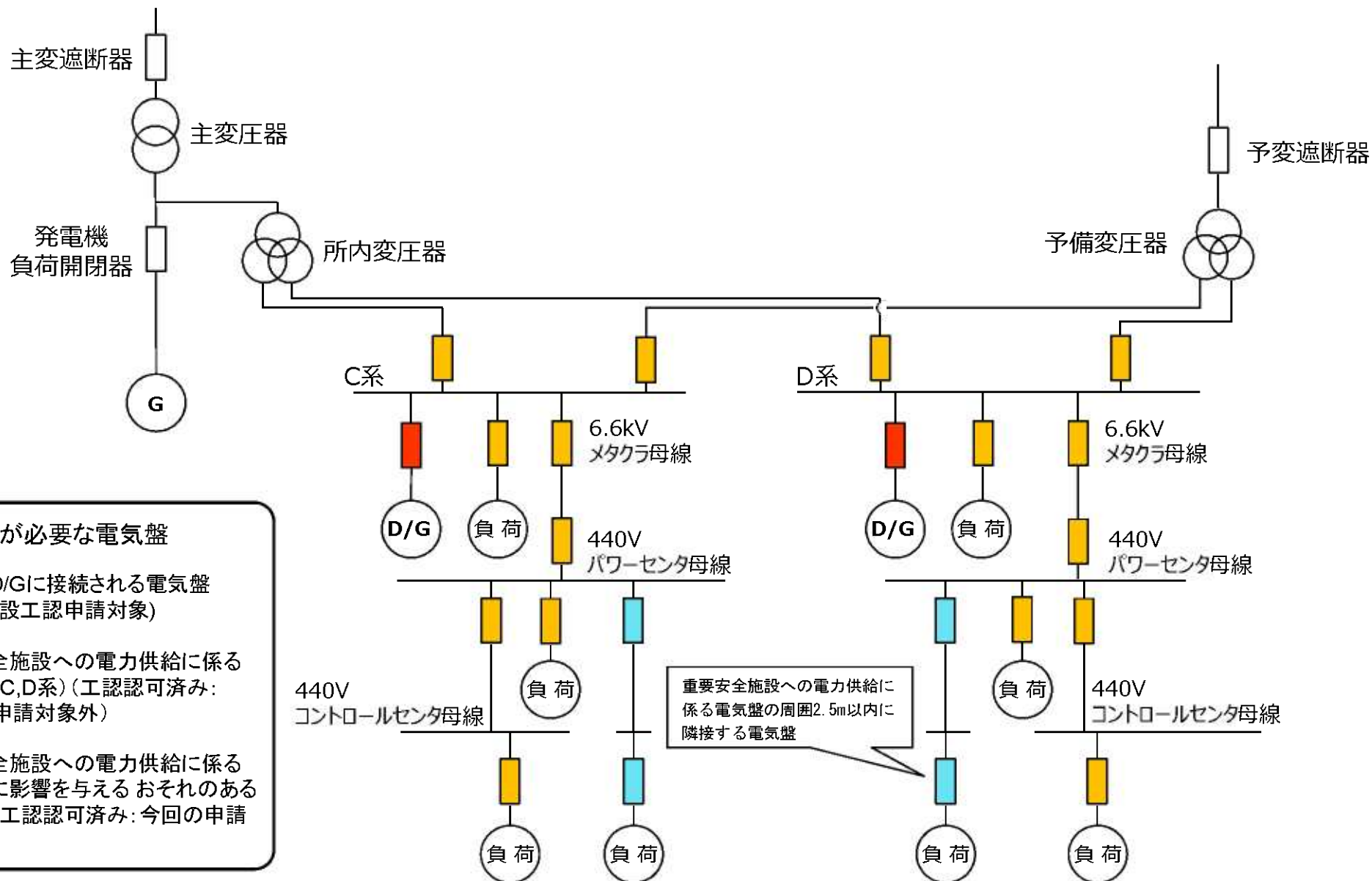
玄海3号機 所内電気系統(概要図) ※玄海4号機も同様
