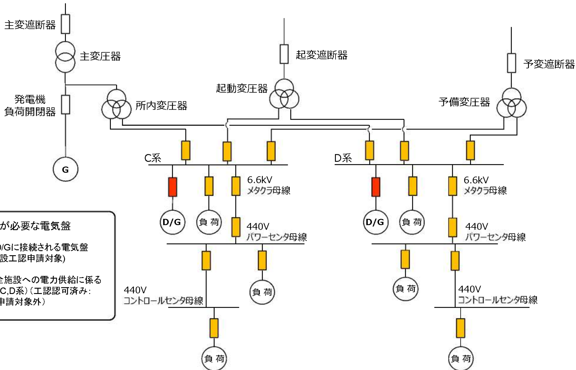
川内1号機 所内電気系統(概要図) ※川内2号機も同様
