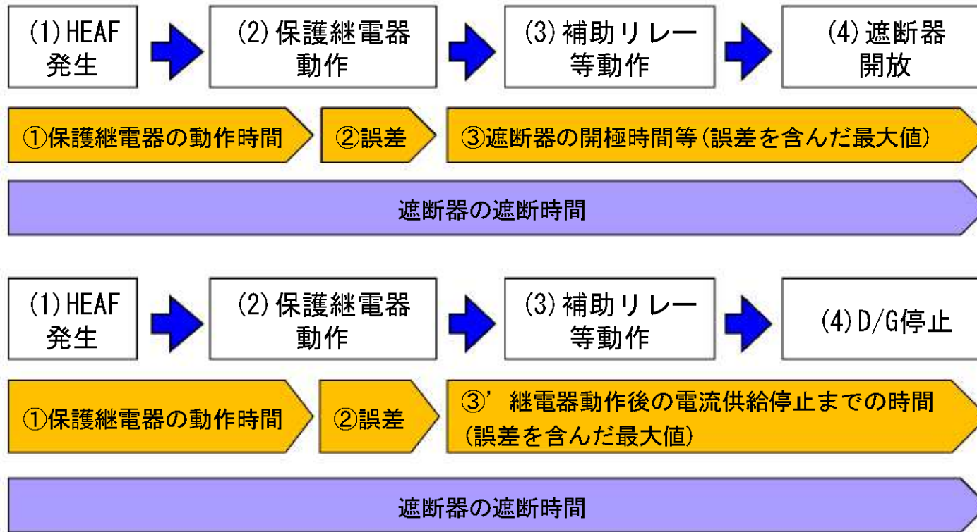
図1 遮断器の遮断時間に含まれる誤差の考え方
