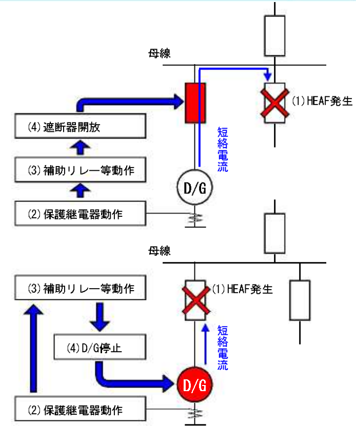
図2 遮断器開放までの流れ
