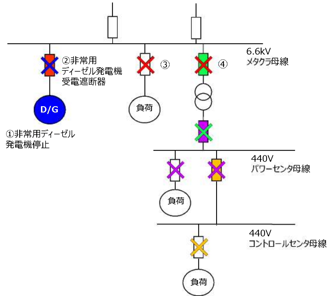
所内電気系統（概要図）※全プラント共通
