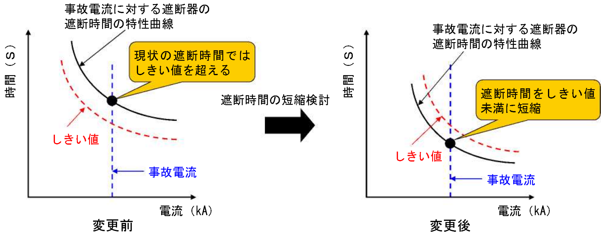
遮断器の遮断時間変更イメージ図
