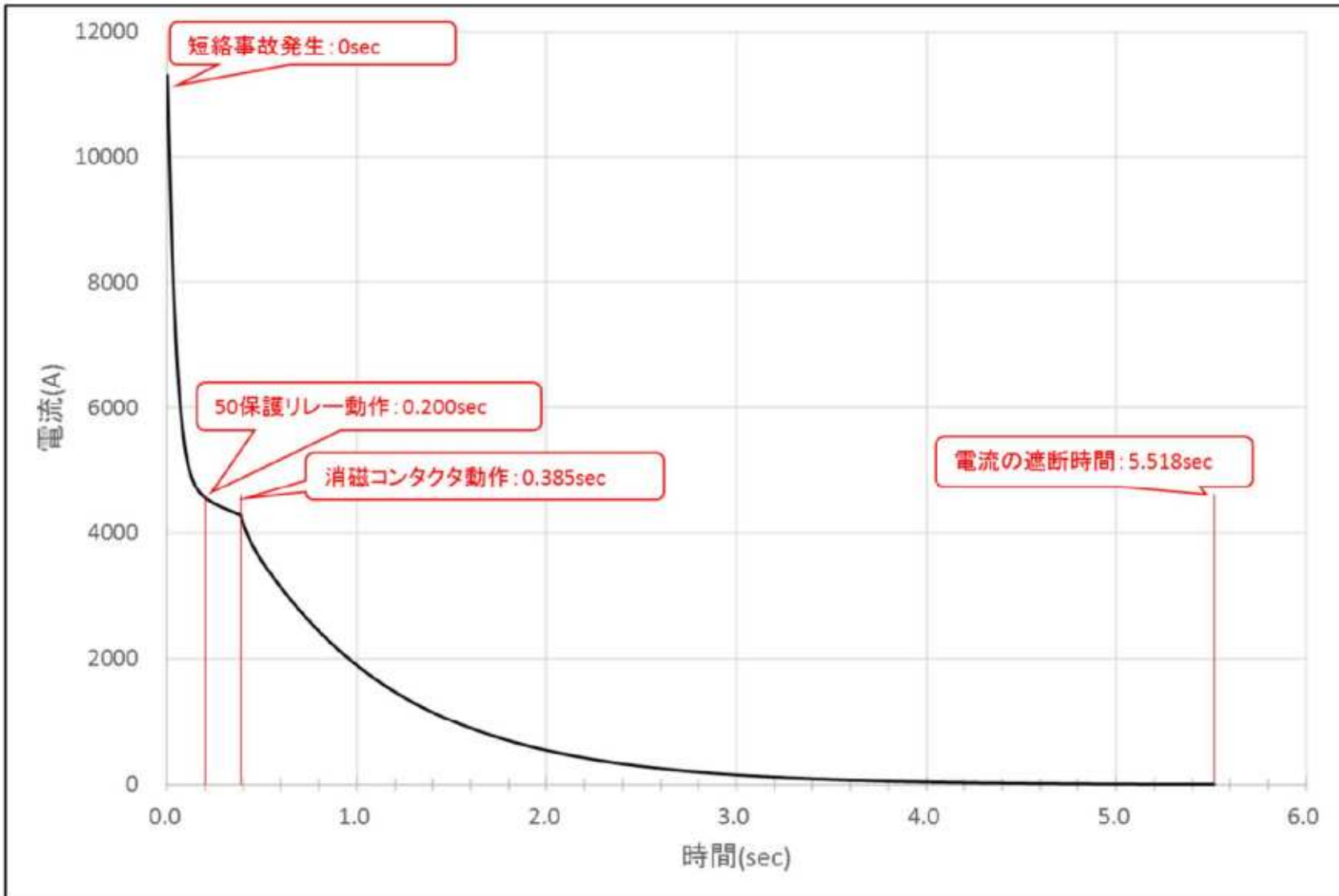
非常用ディーゼル発電機受電遮断器においてHEAFが発生した場合の アーク電流の減衰(玄海3/4号機)
