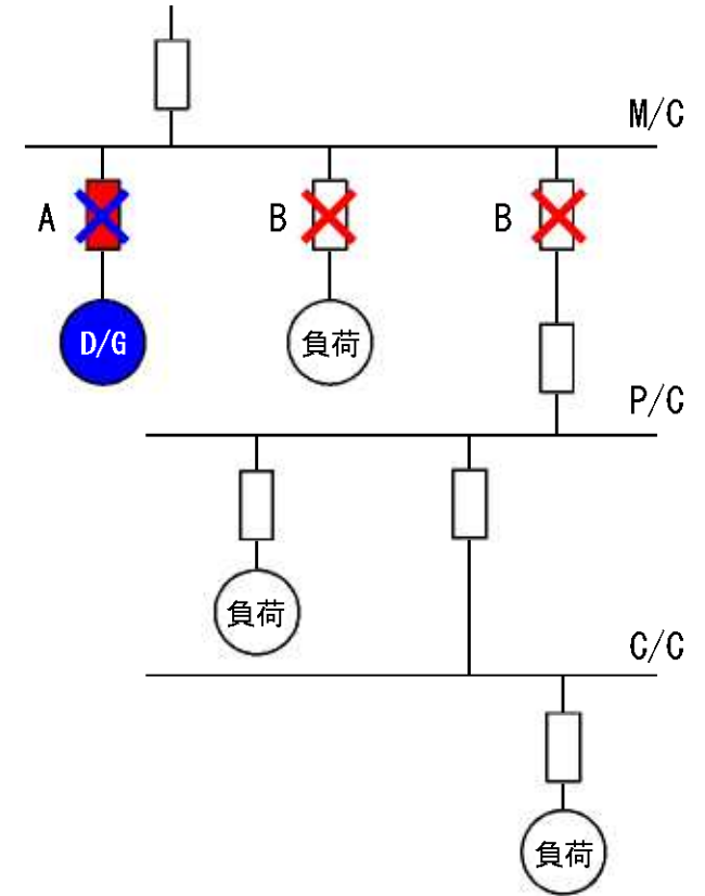
所内電気系統 (概略図) ※全プラント共通
