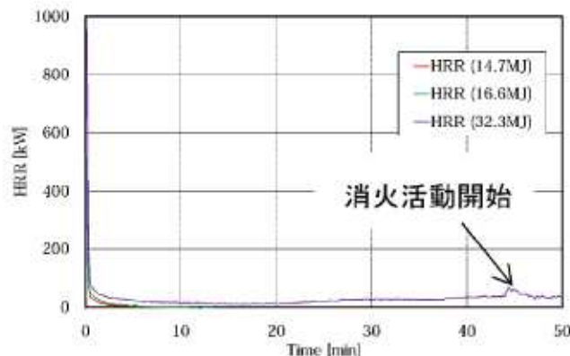
発熱速度(HRR)測定結果(M/C(D/G)試験時)
