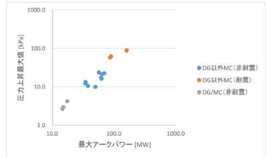
最大アークパワーと圧力上昇最大値の関係
