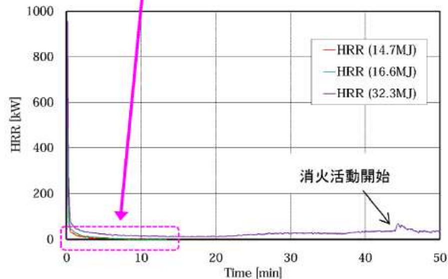
発熱速度(HRR)測定結果(M/C(D/G)試験時)
