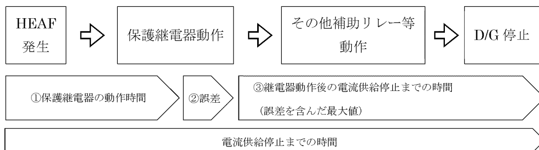
図 6.2.2 電流の供給停止時間に含まれる誤差の考え方 (非常用ディーゼル発電機に接続される電気盤)
