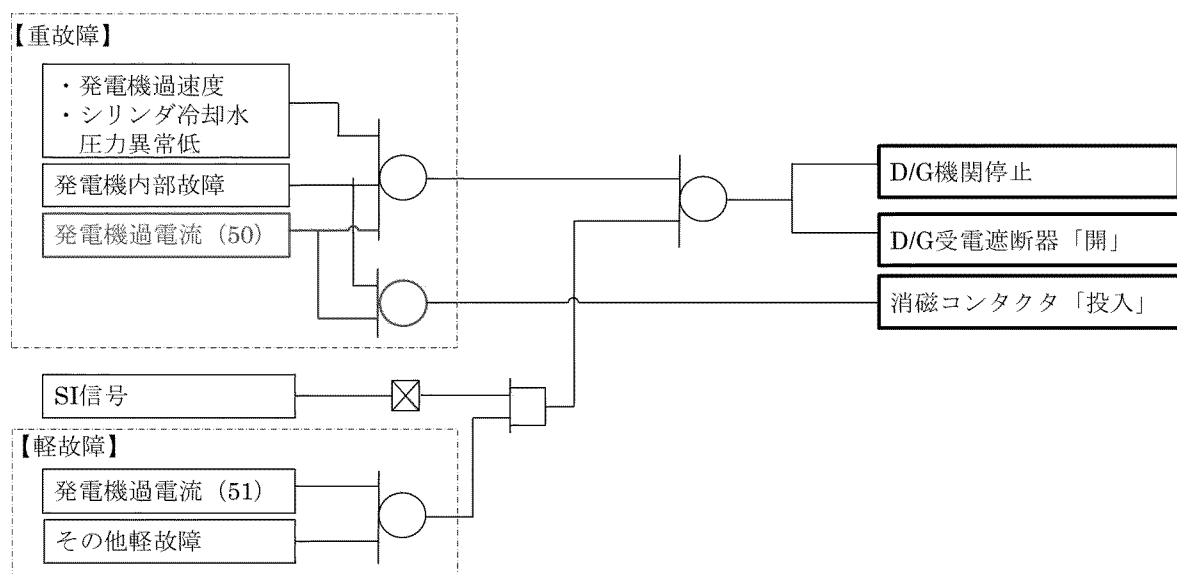
図 6.4 インターロック図（概要）
