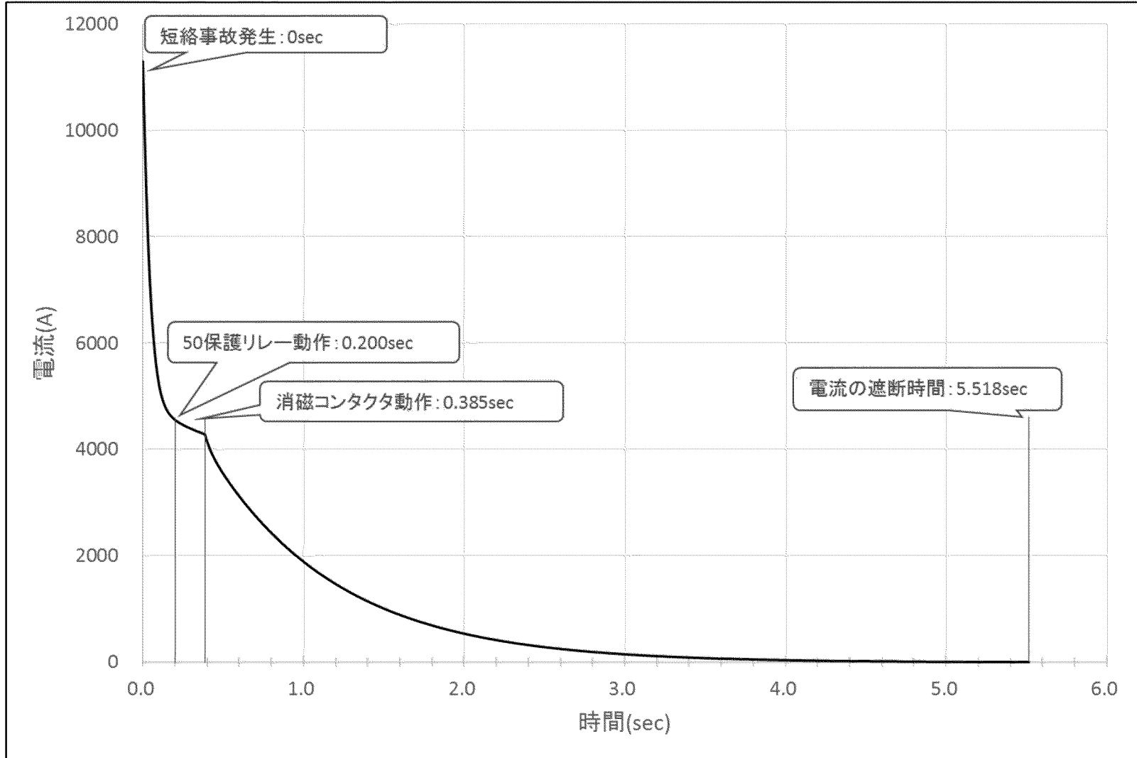
図 6.3 アーク電流の減衰（玄海 3 号機）
