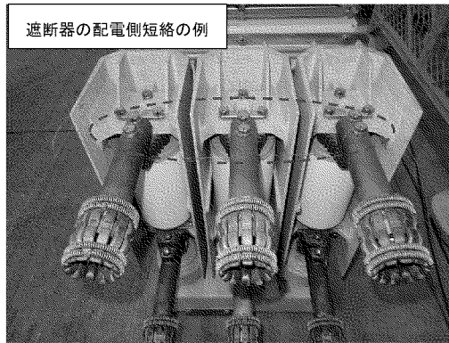
図 4.5.4 遮断器の短絡箇所 (M/C (D/G) 試験時) (非常用ディーゼル発電機に接続される電気盤)
