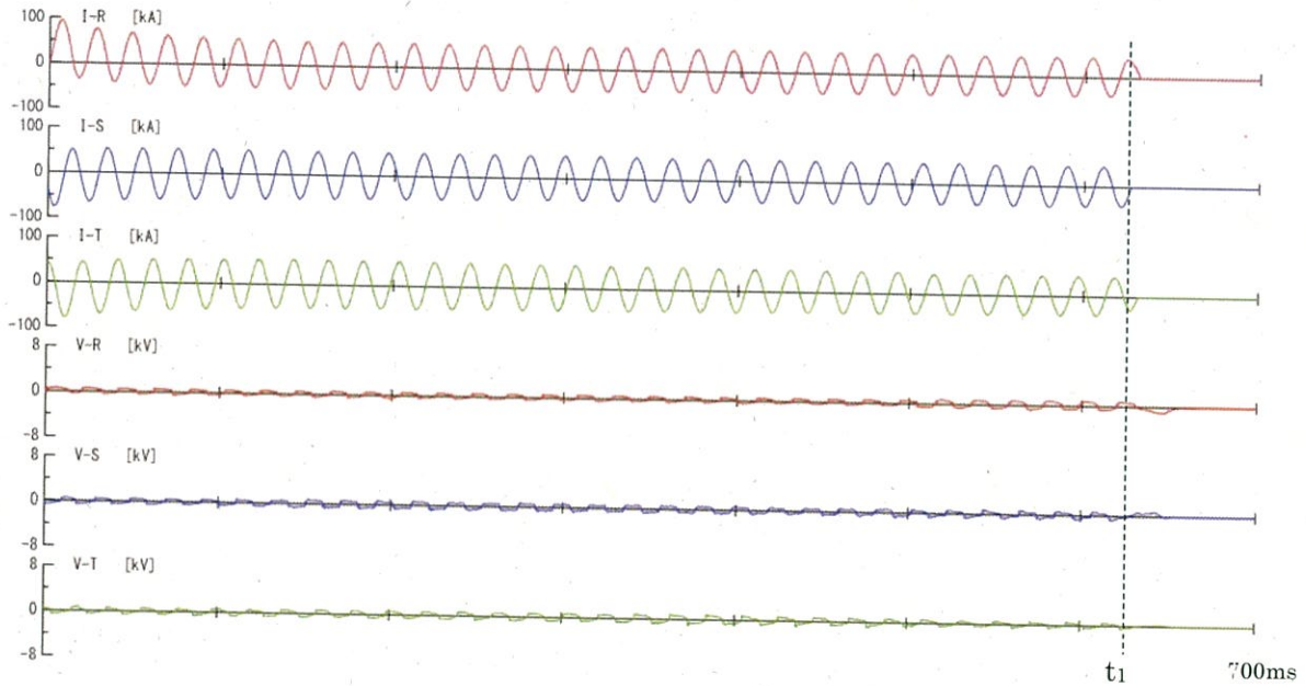
図 4.7.1 HEAF 試験時の電圧・電流波形 (M/C)
