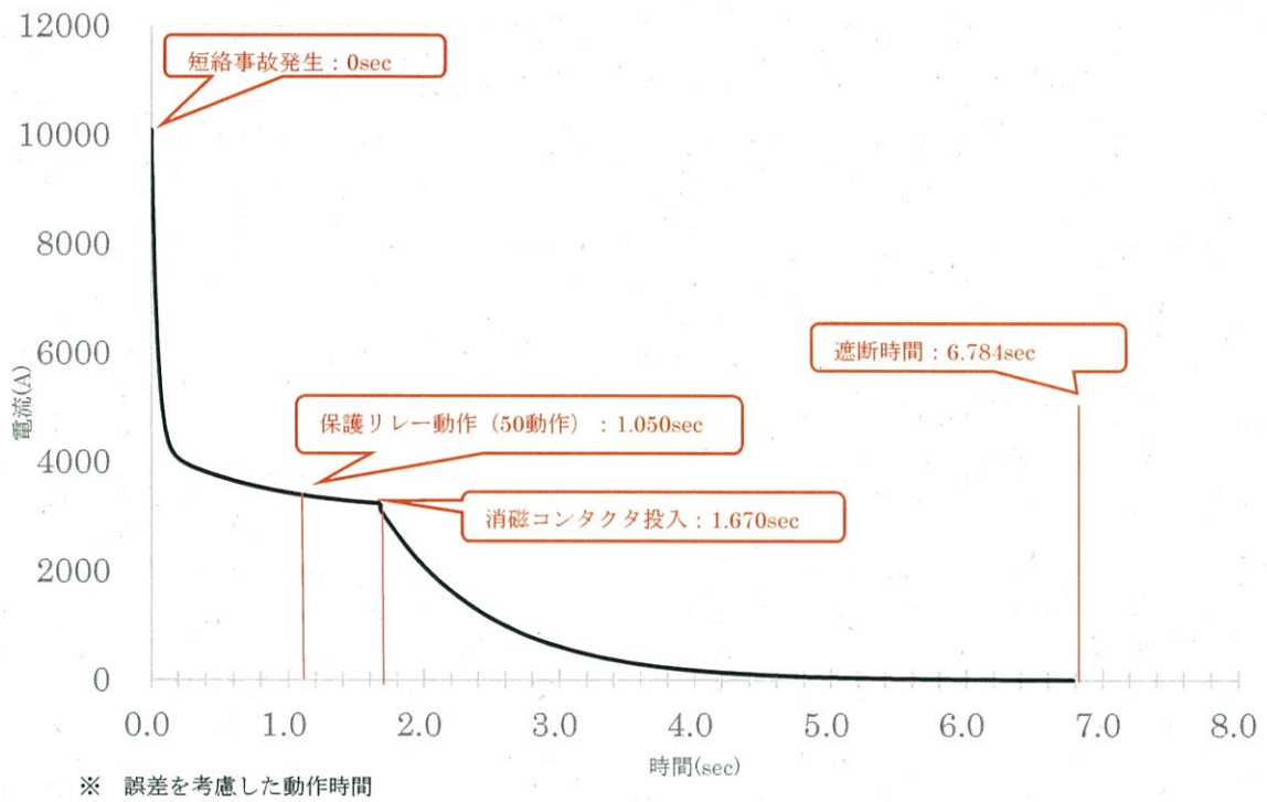
図 6.3 アーク電流の減衰 (伊方 3 号機)
