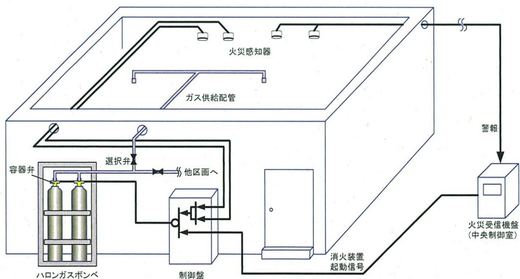
図 6.5 火災感知設備及び消火設備のシステム構成概要図
