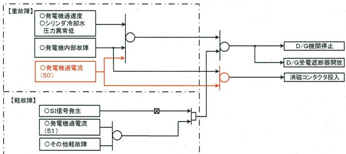
図 6.3 インターロック図 (概要)
