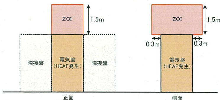
図 6.6 火災感知器に対する HEAF の ZOI
