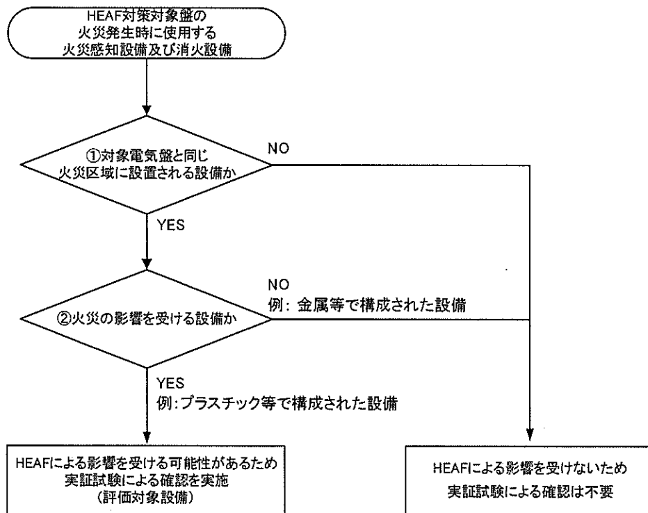
図 6.4 評価対象設備の選定フロー
