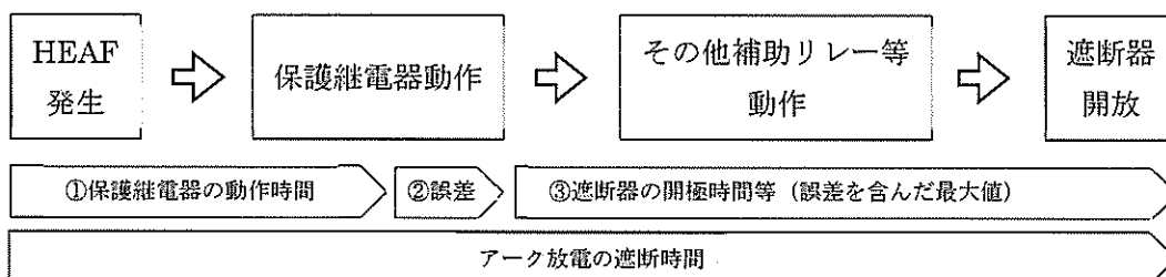
図 6.2.1 遮断器の遮断時間に含まれる誤差の考え方
