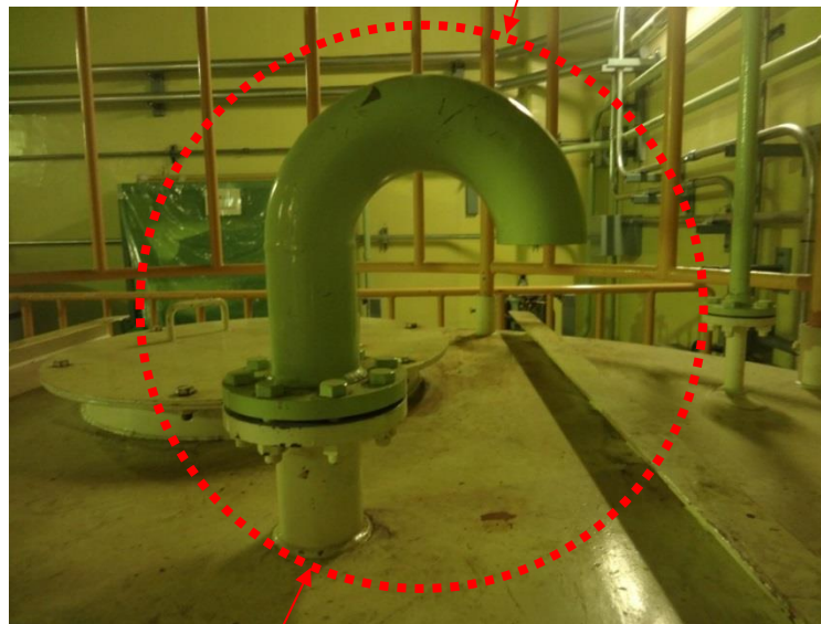
B-原子炉補機冷却系サージタンクのベント管
