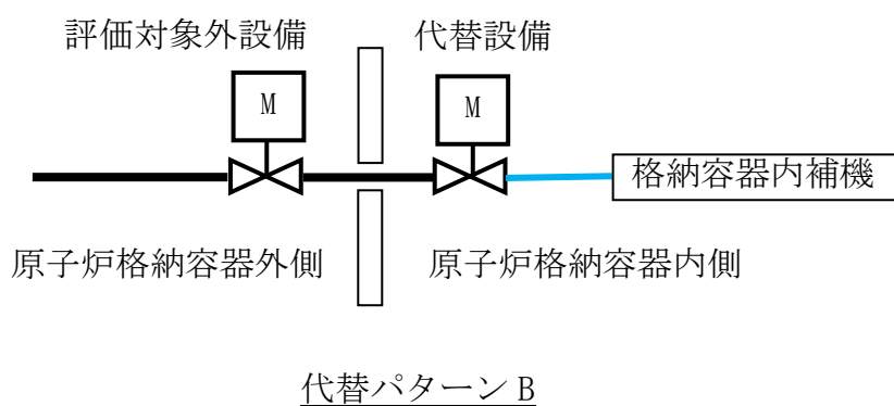
図 2-5 系統概略図
