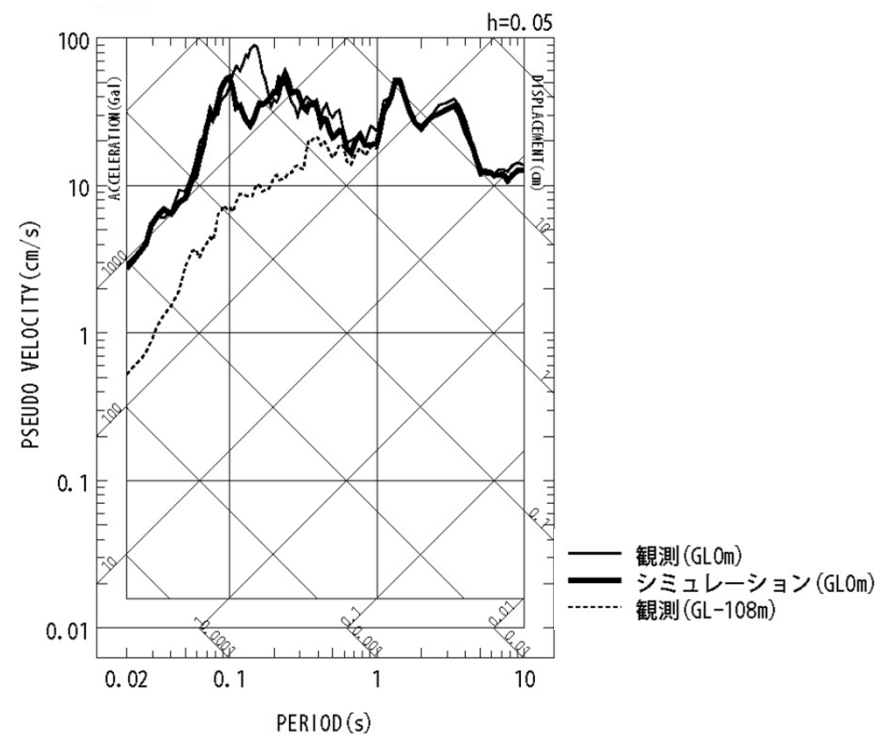
UD 応答スペクトルの比較(鉛直)
