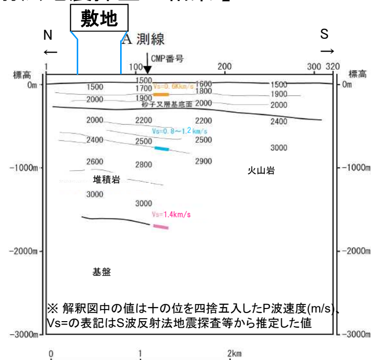
C測線深度断面
