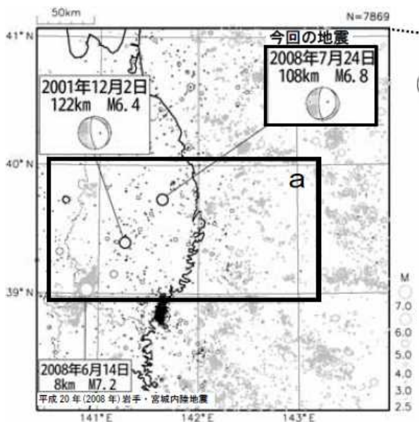
図2-1 震央分布図
