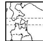
東西断面図(北緯:41.5° ~41.7° ) (1997年10月～2014年3月)
