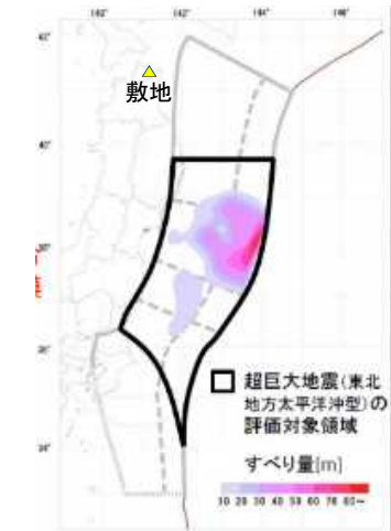
地震調査委員会(2019)による超巨大地震の震源領域 ※ 地震調査委員会(2019)より転載・一部加筆
