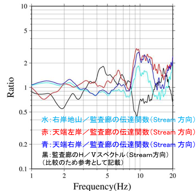
伝達関数
