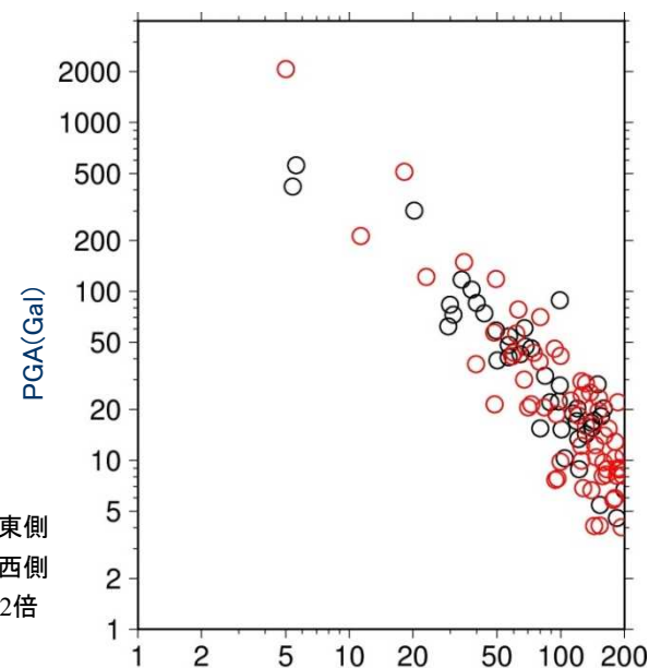
断層最短距離(km) 最大加速度分布
