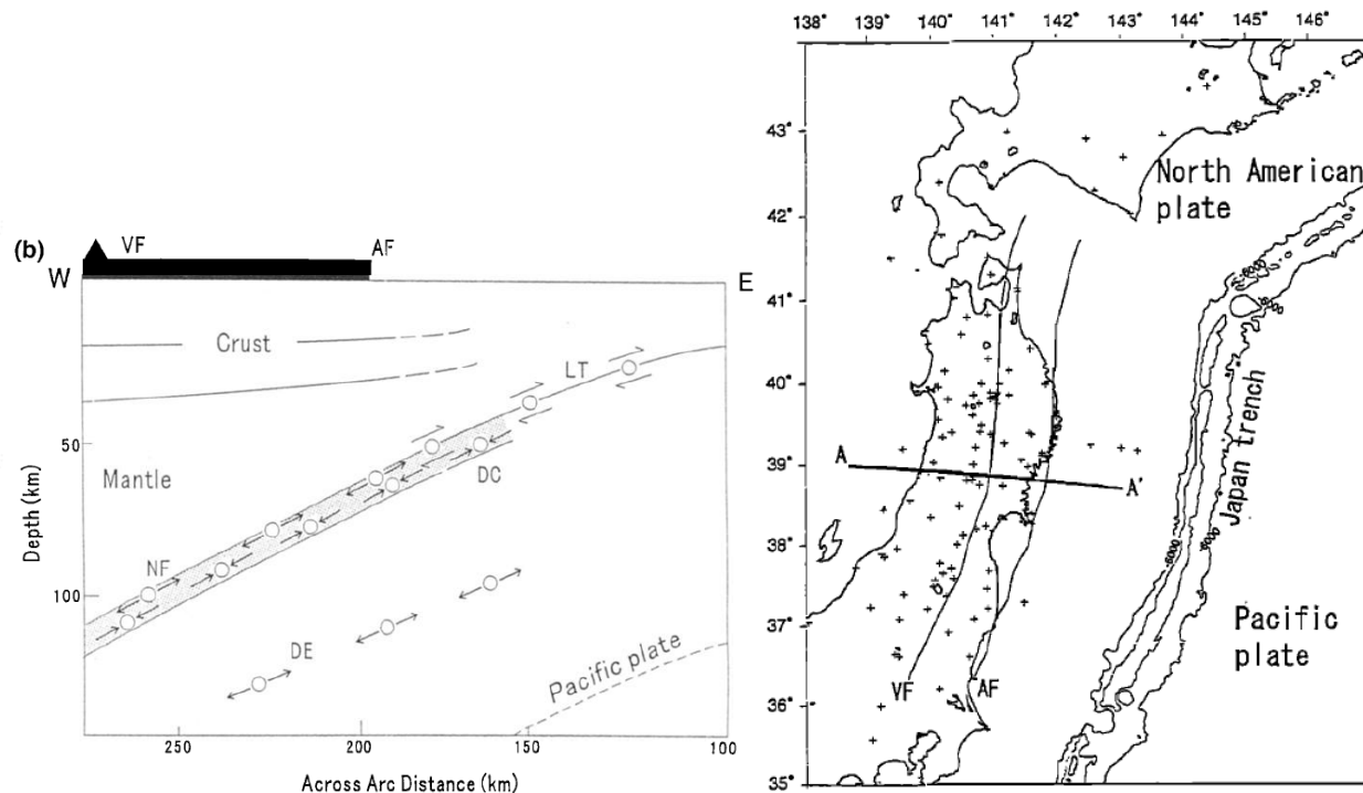
Igarashi et al.(2001)によるアサイズミックフロント位置 (図中AF:アサイズミックフロント、LT:プレート間地震)
