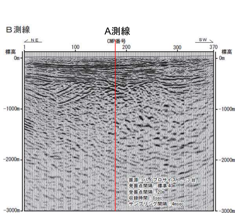
B測線深度断面
