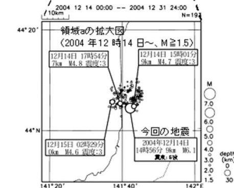
2004年北海道留萌支庁南部地震および周辺で発生した主な地震
