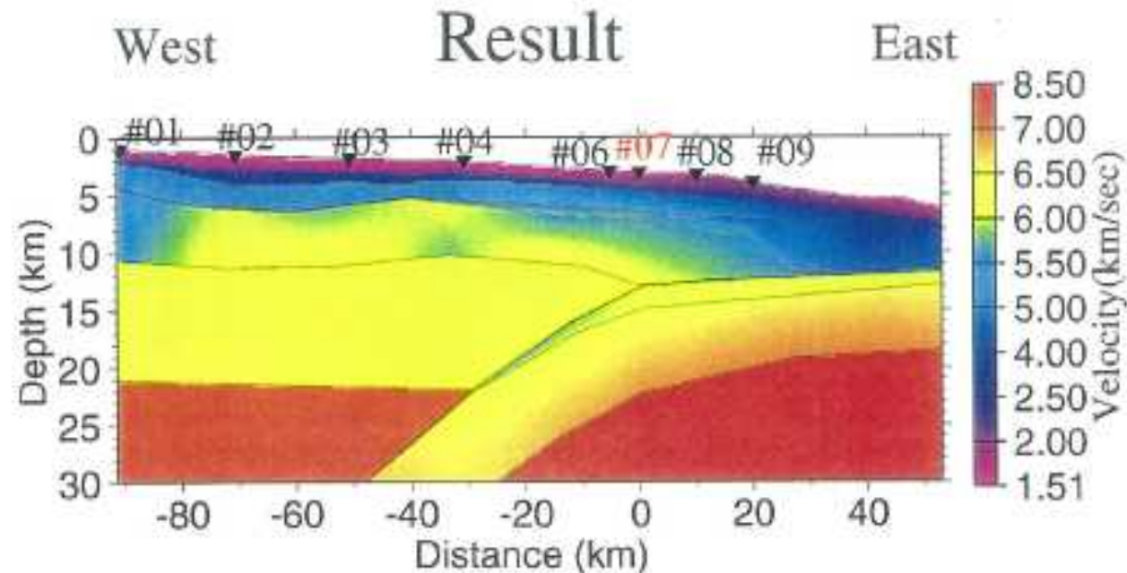
Figure 6.6: 東西測線の構造。走時インバージョンの結果。 藤江(1999)より抜粋
