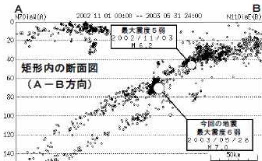
図2-1 震央分布図、断层面図
