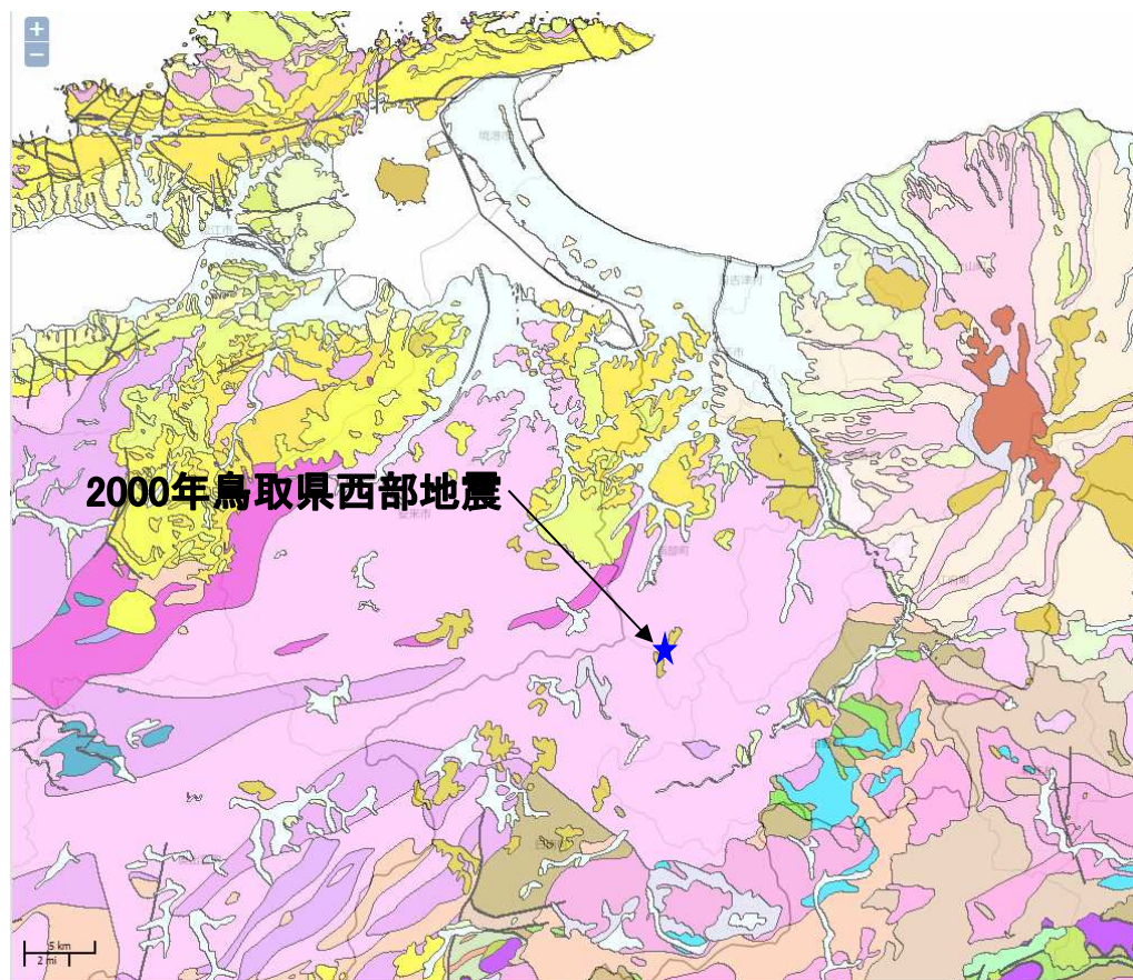
シームレス地質図
