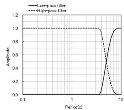
破壊開始点2,4
