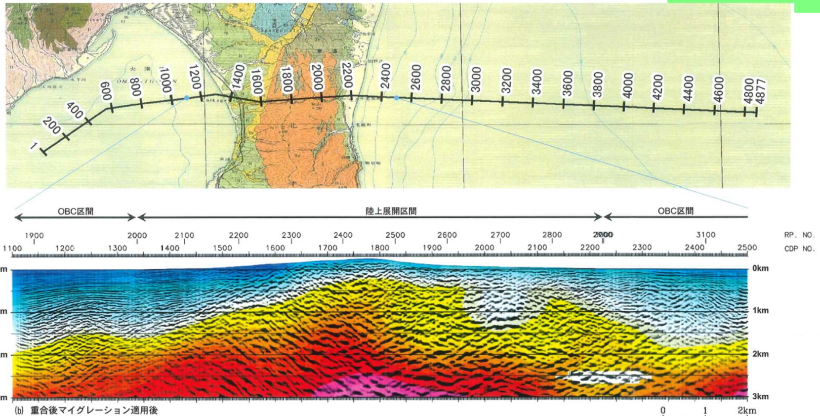
反射法・屈折法統合深度プロフィール[3]下北半島横断陸域－浅海域区間(V:H = 1:1)
