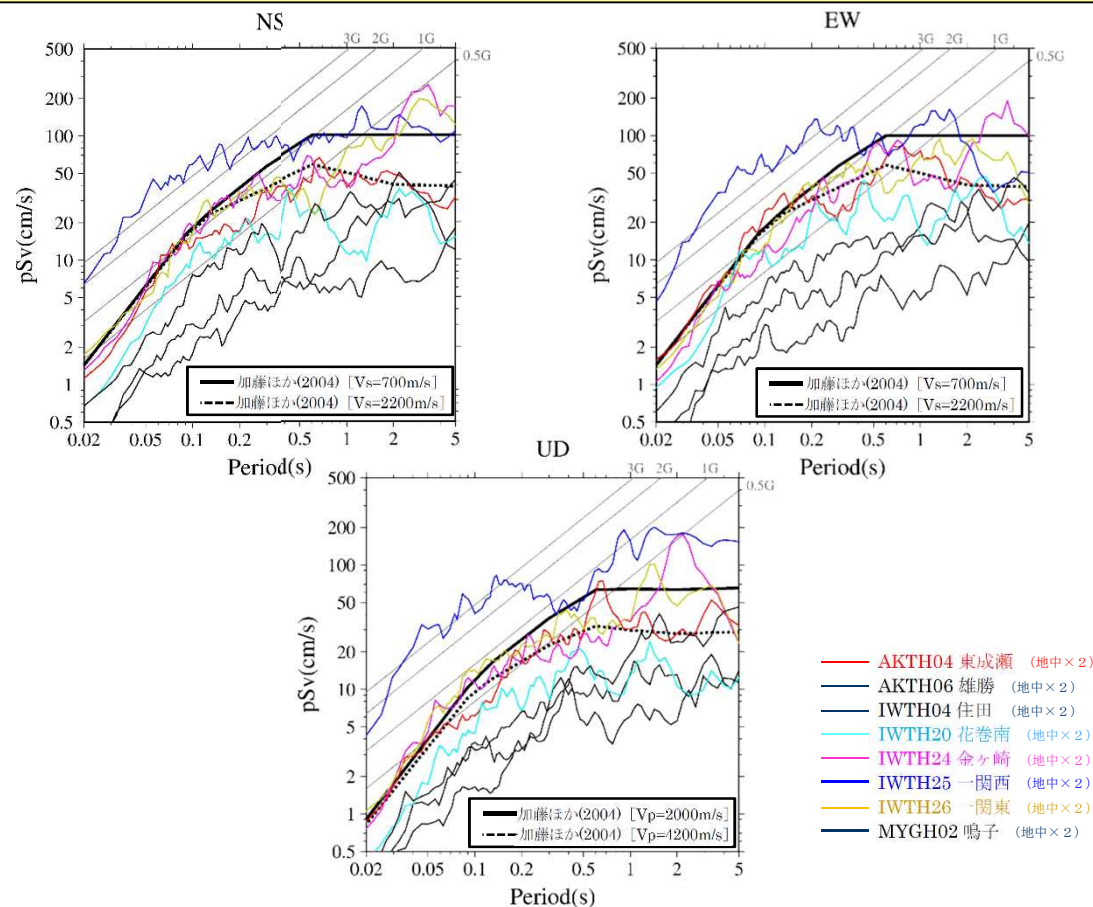
KiK-net観測記録の応答スペクトルと加藤ほか(2004)による応答スペクトルの比較
