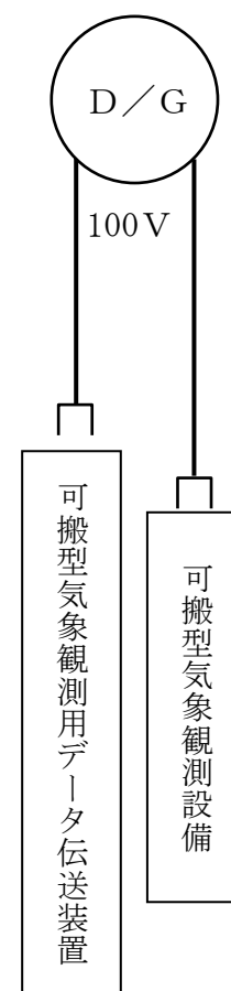
第 33. 6 図 可搬型発電機接続時の系統図
