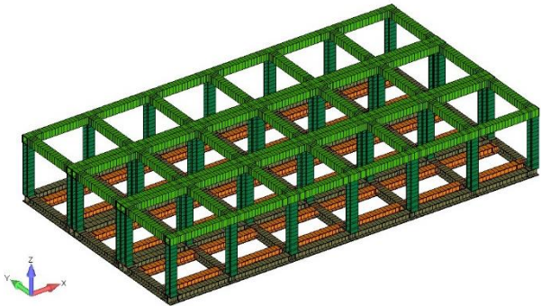
使用済吸着塔保管架台のみの 地震応答解析モデル
