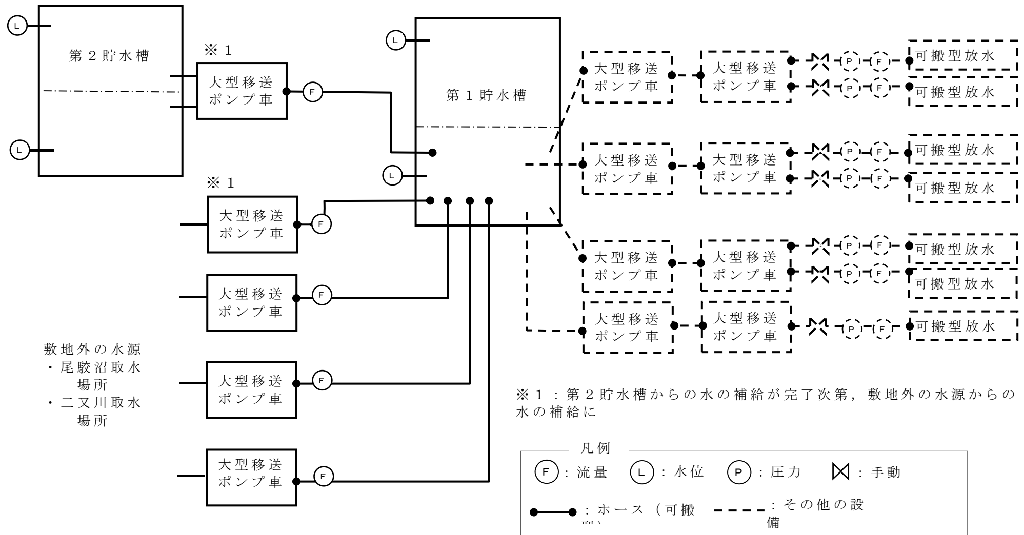
第 4 図 重大事故等への対処に必要となる水の供給設備の系統概要図 (その 1) (大気中への放射性物質の拡散抑制への対処及び第 1 貯水槽へ水を補給の対処)
