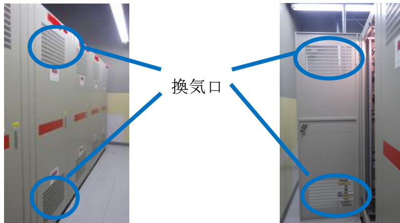
第3図 再処理施設の安全系制御盤（換気ファン無し）
