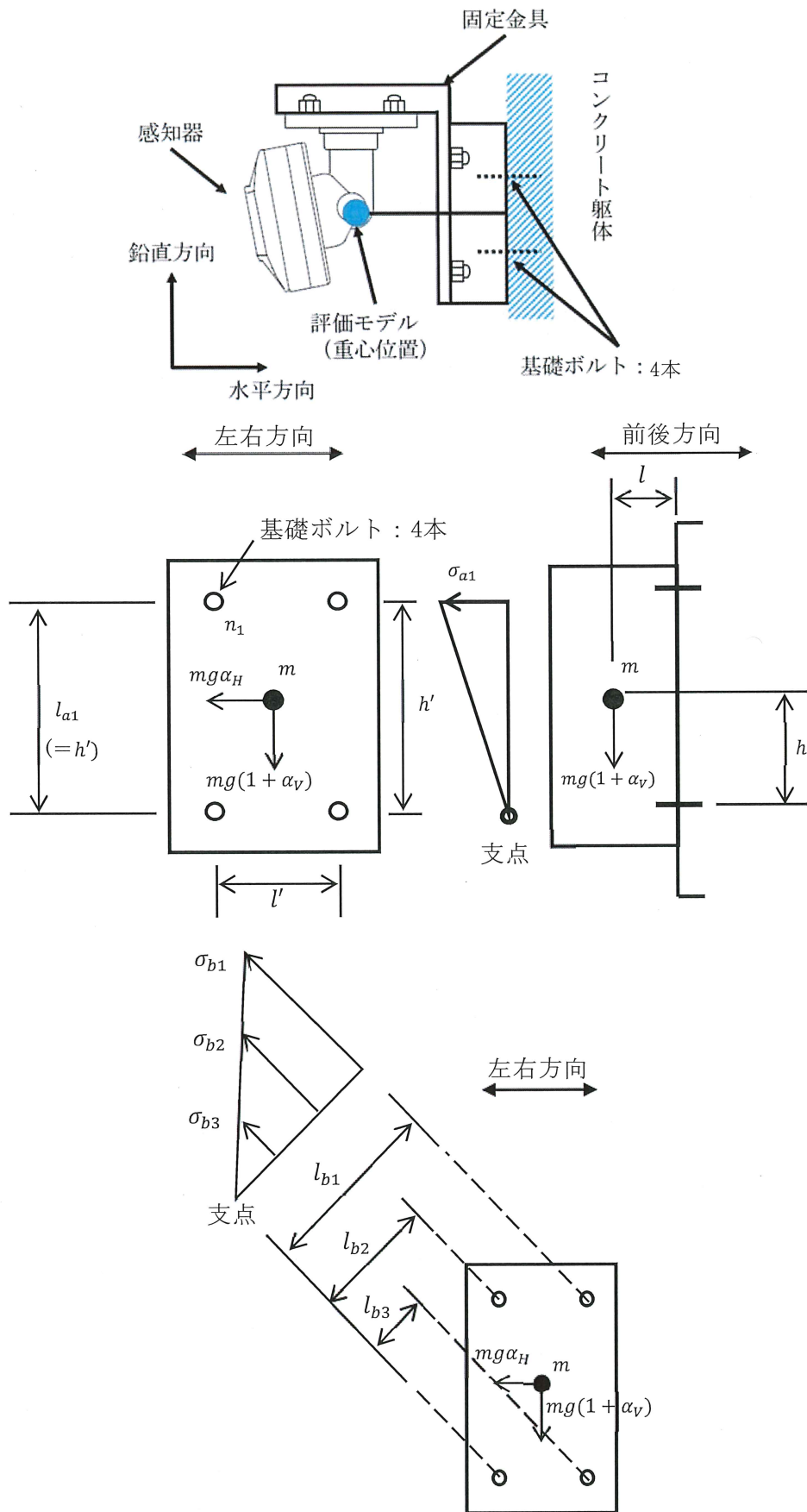
第5-3図 四点固定型（壁掛け型）の応力評価モデル（左右方向）
