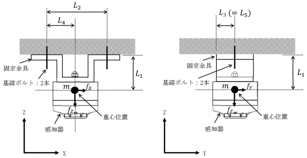
第5-1図 二点固定型（天井支持型）の応力評価モデル
