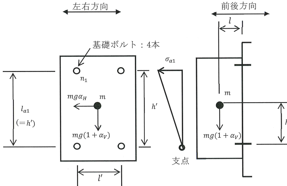
第5-2図 四点固定型（壁掛け型）の応力評価モデル（前後方向）
