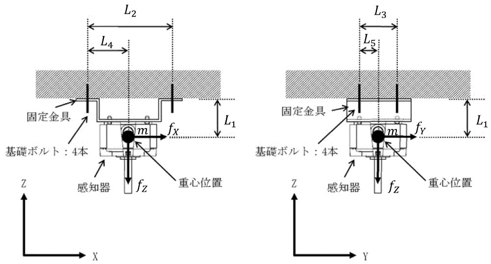
第5-4図 四点固定型（天井支持型）の応力評価モデル
