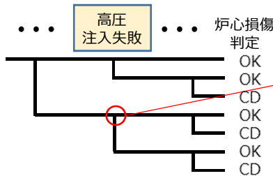
緩和系ET（小破断LOCA）（概念図）
