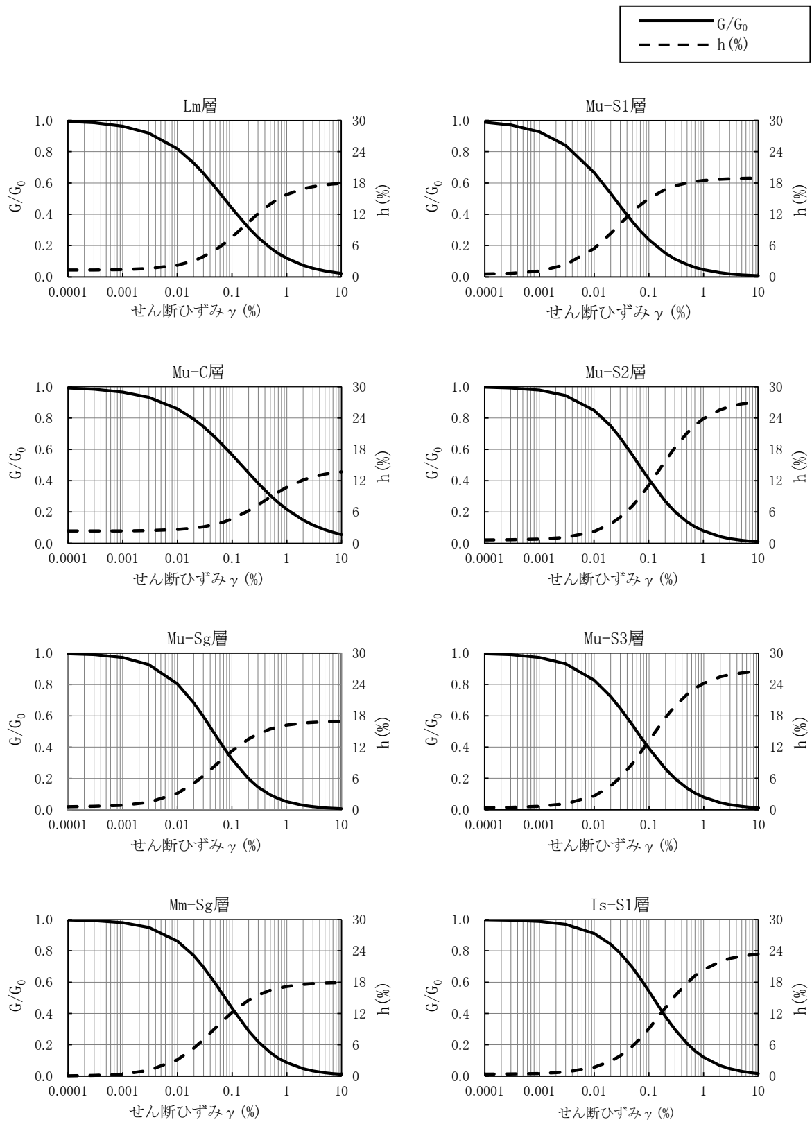
図 2-1 地盤の非線形特性(1/2)
