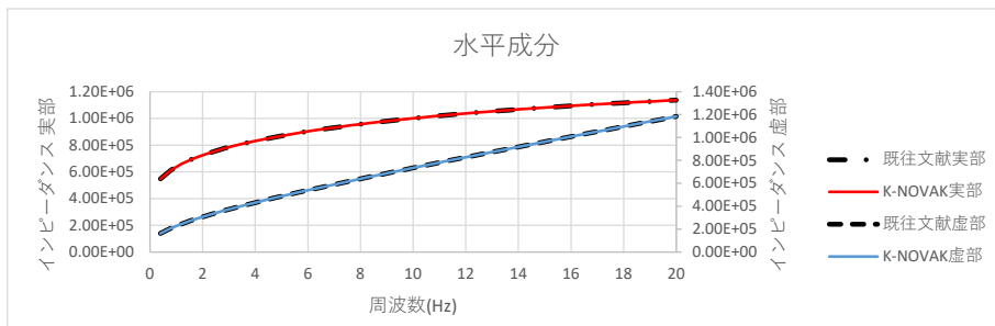
図 2-5 計算結果比較 (水平ばね)
