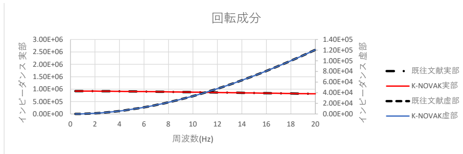
図 2-6 計算結果比較 (回転ばね)
