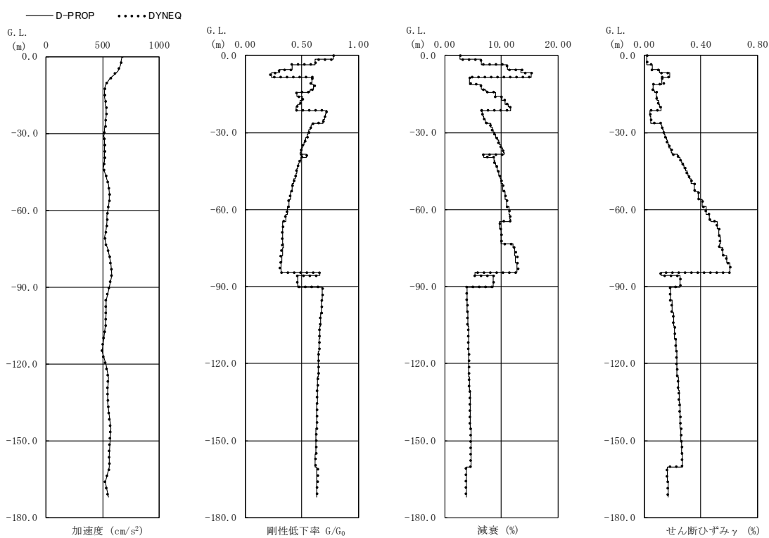
図 2-4 地盤の地震応答解析結果の比較 (Ss-D, 水平方向)
