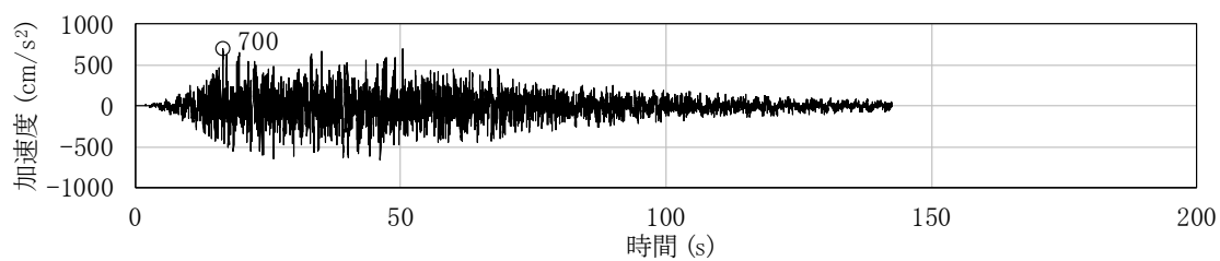
図 2-3 基準地震動の時刻歴波形 (Ss-D, 水平方向)
