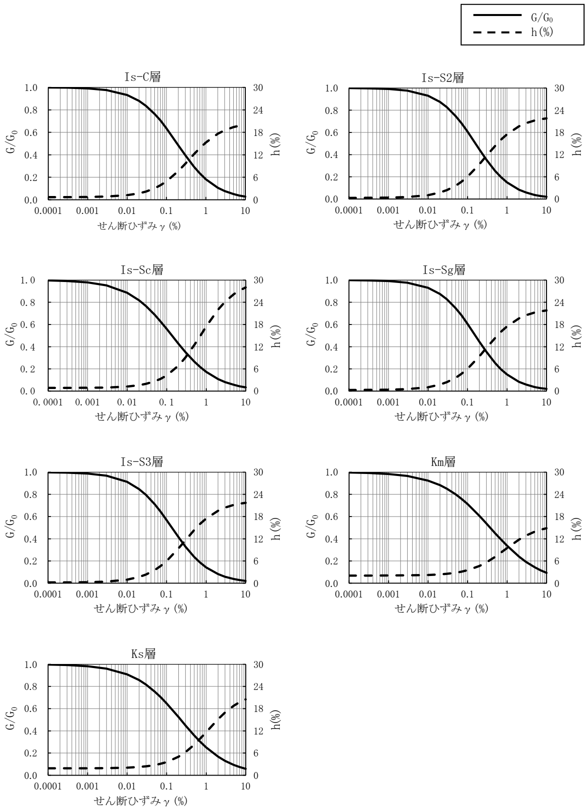
図 2-2 地盤の非線形特性 (2/2)
