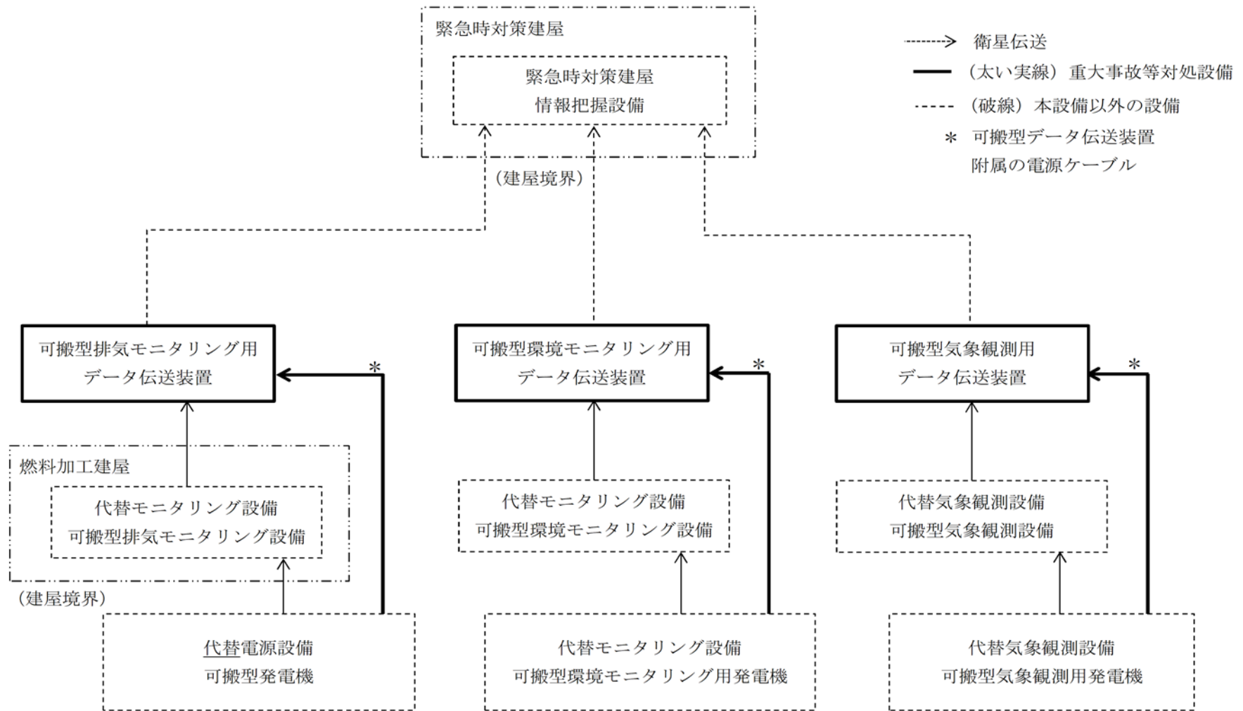
第4図 可搬型排気モニタリング用データ伝送装置の系統概要図
