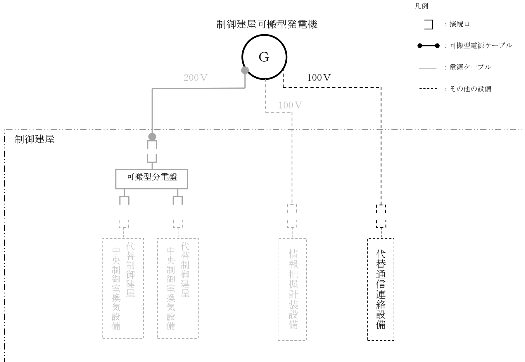
第 2.1.7.3-5 図 系統図 (制御建屋可搬型発電機)
