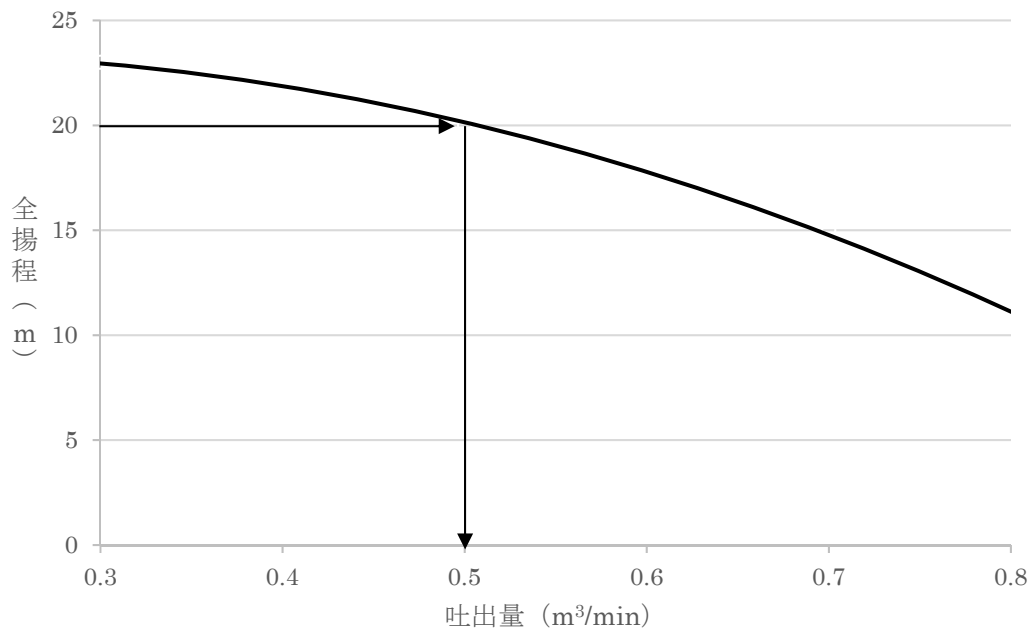
図3 可搬型排水ポンプ性能曲線 (例)
