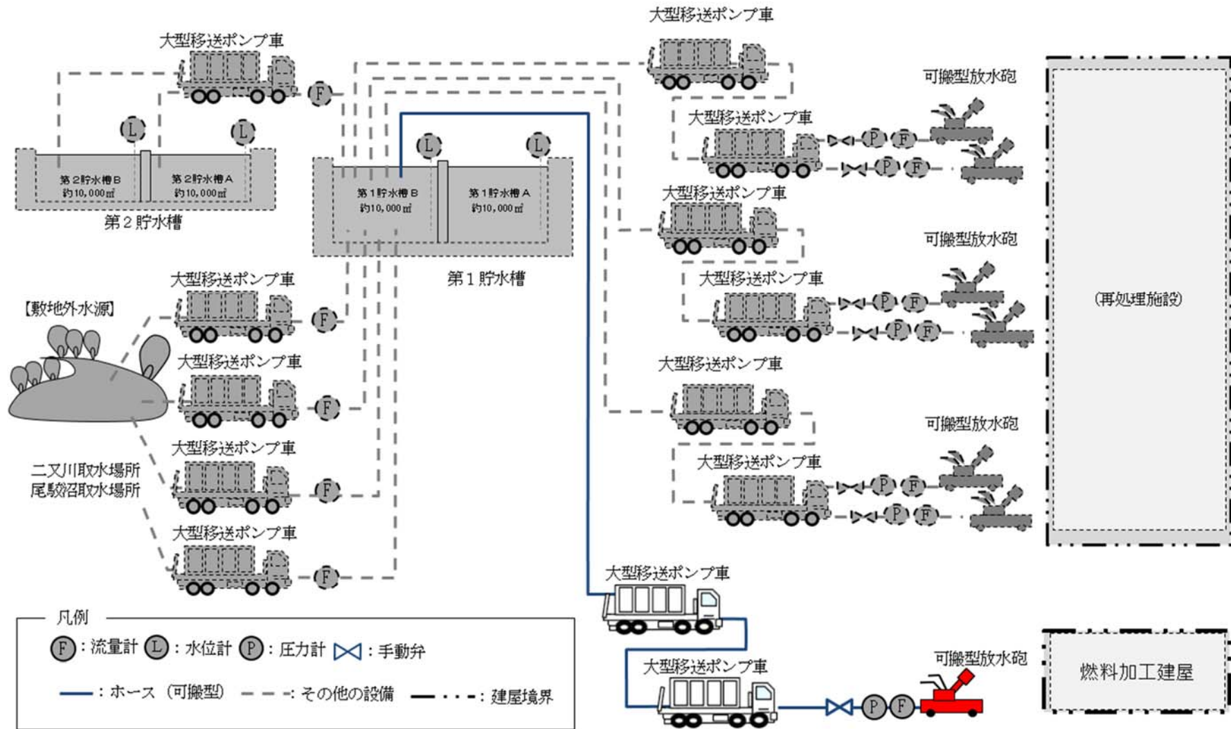
図1 工場等外への放射性物質の拡散を抑制するための設備の系統概要図 (その1) (大気中への放射性物質の拡散抑制)
