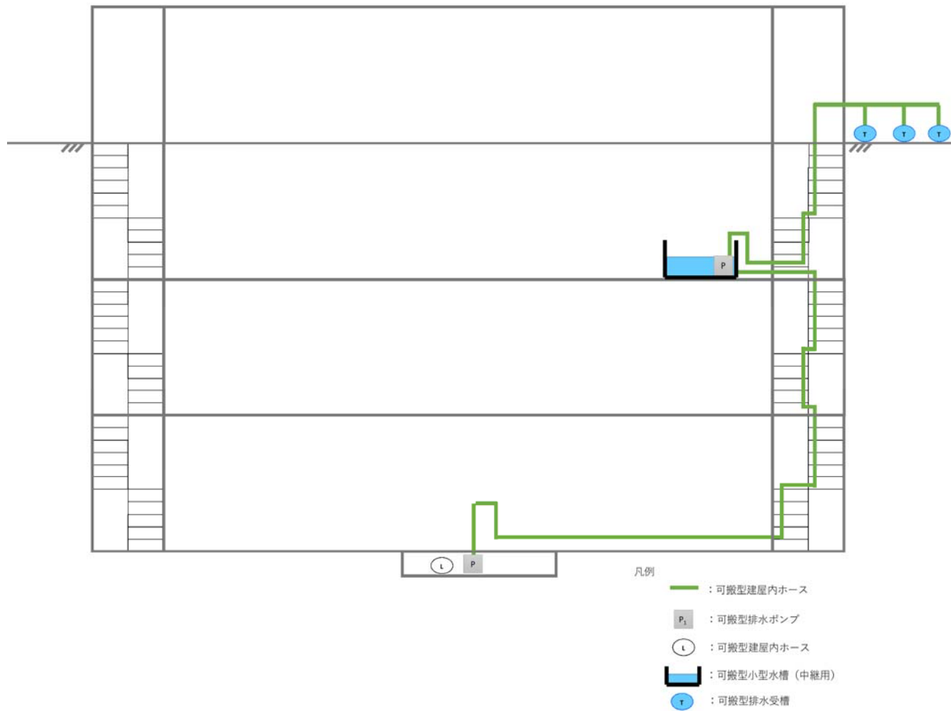
図3 工場等外への放射性物質の拡散を抑制するための設備の系統概要図 (その3) (燃料加工建屋からの排水)
