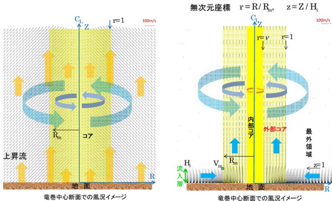
第6-1図 風速場モデル
