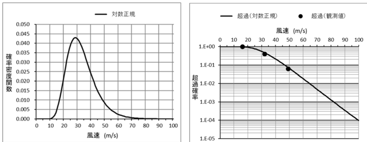
添3-11 風速の確率密度分布（左）と超過確率（右）
