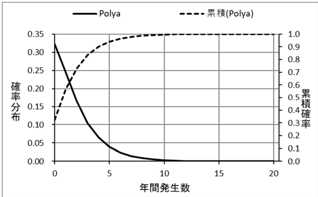
添3-10 竜巻検討地域における竜巻発生数の確率分布と累積確率
