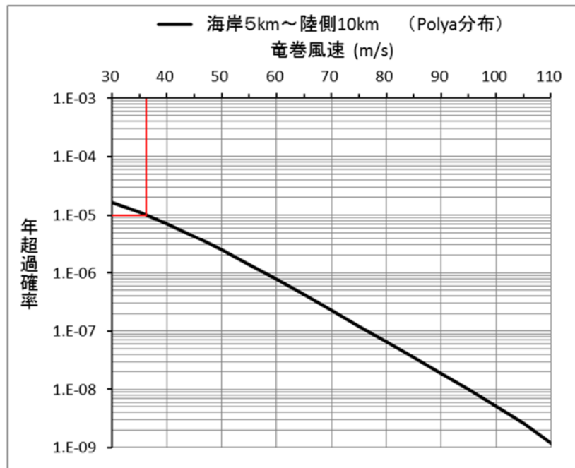
(a) 竜巻最大風速のハザード曲線
