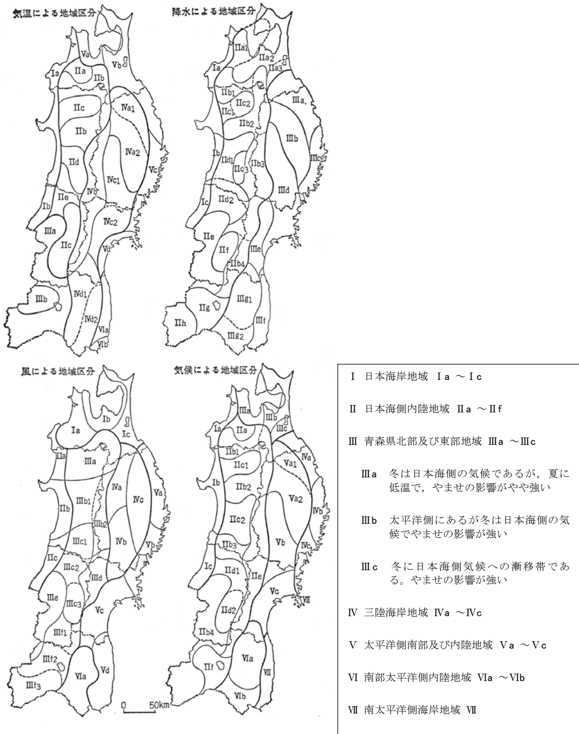
添3-1第1図 吉野正敏（1967年から）による東北地方の気候区分
