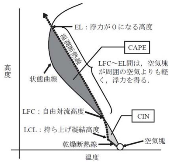
添3-千第6図 CAPEの概念
