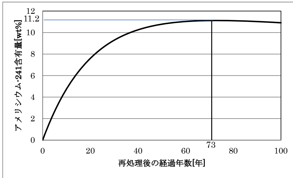
第 3.2.1 図 再処理後の経過年数に対するアメリシウム-241 含有量の推移
