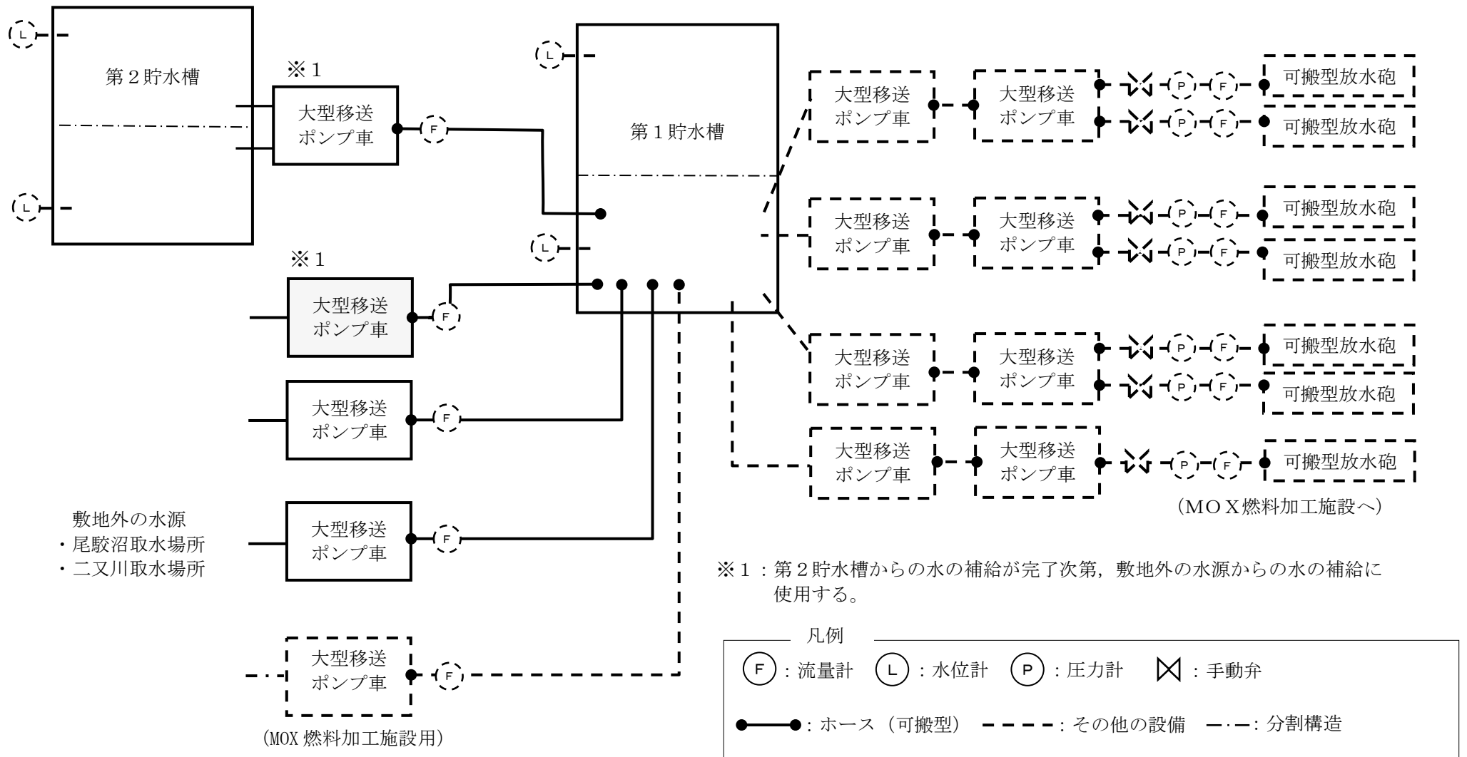
第9.4-4図 水供給設備の系統概要図 (大気中への放射性物質の放出抑制への対処に係る第1貯水槽への水の補給)
