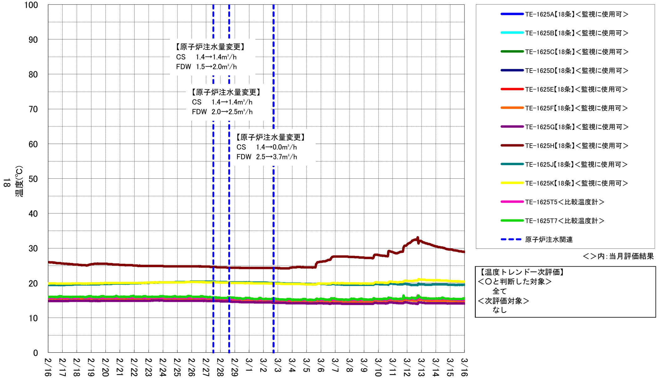
1号機 実施計画関連温度計(PCV)
