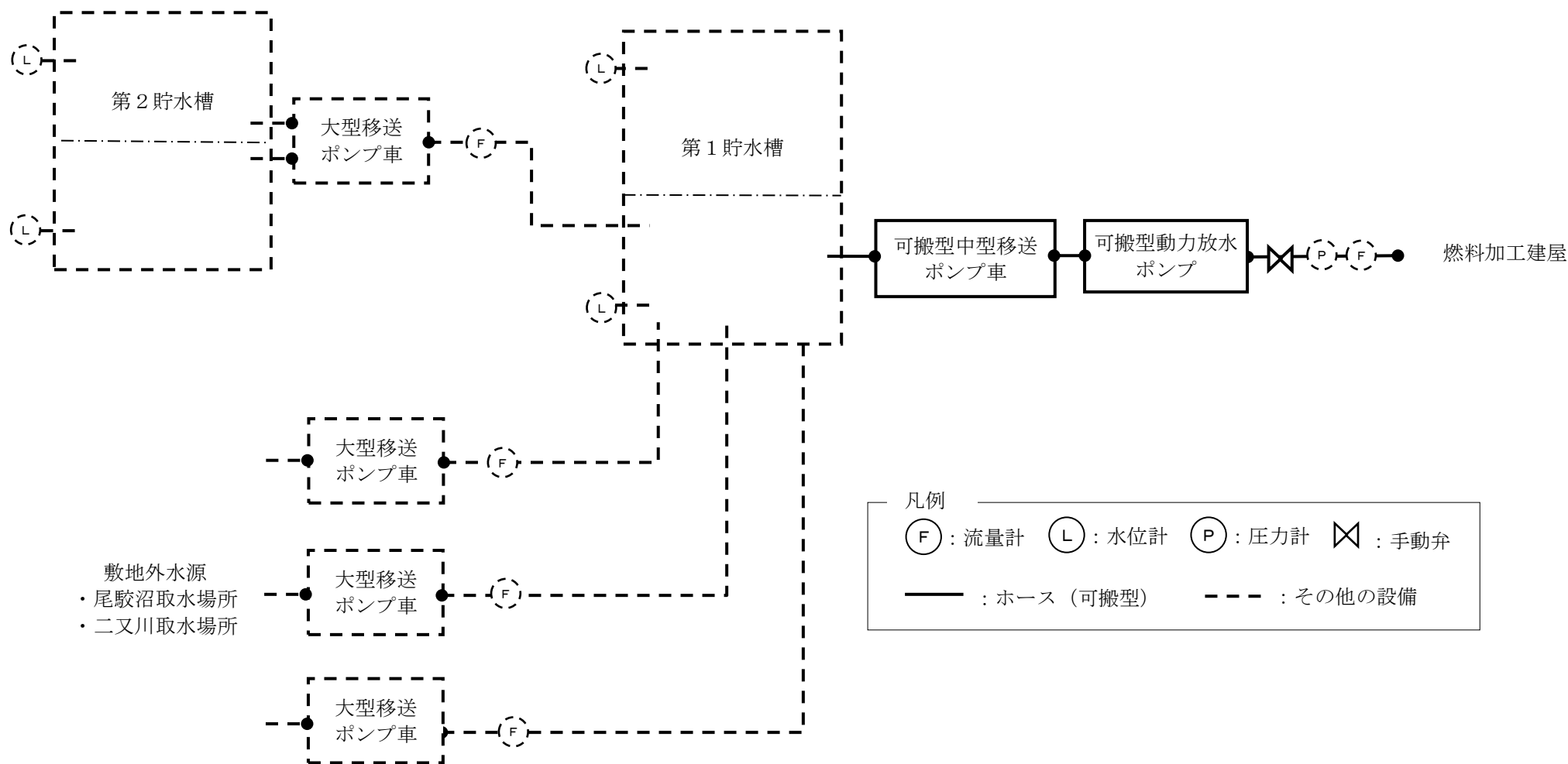
第 30. 1 図 工場等外への放射性物質の拡散を抑制するための設備の系統概要図 (その 1) (大気中への放射性物質の拡散を抑制するための設備)
