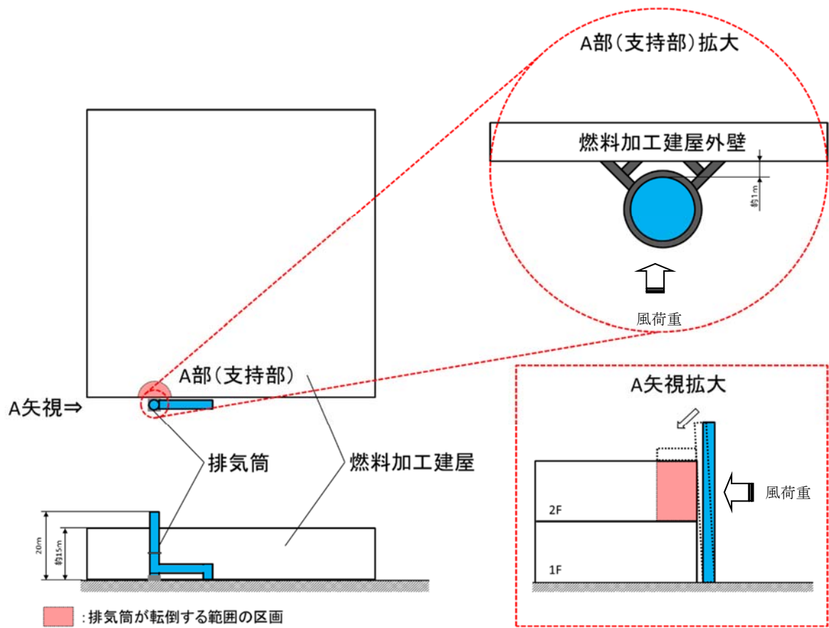
第3-5-1図 燃料加工建屋と気体廃棄物の廃棄設備の排気筒の位置関係
