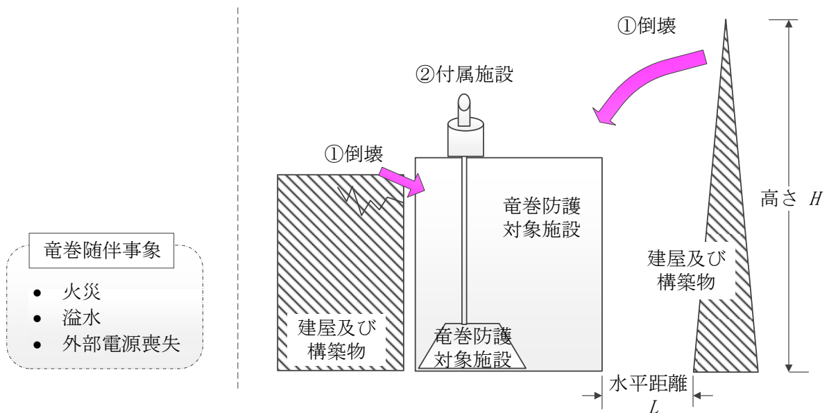
第3-4-2図 竜巻防護対象施設に波及的影響を及ぼし得る
