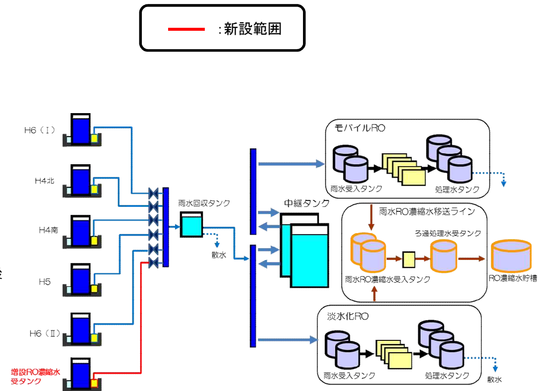
増設RO濃縮水受タンクエリア集水ピット抽出ポンプ新設後
