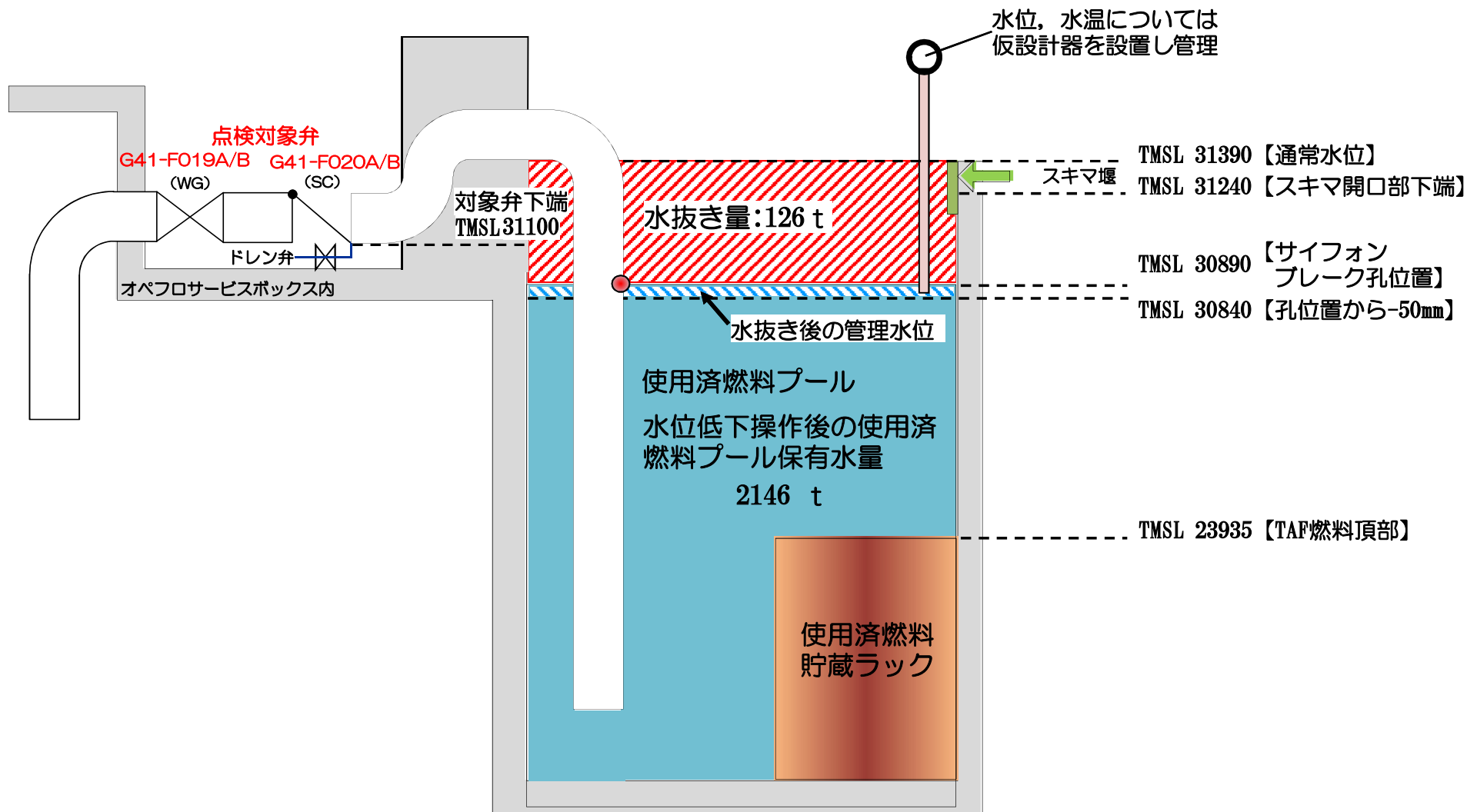
使用済燃料プール弁点検の概略図
