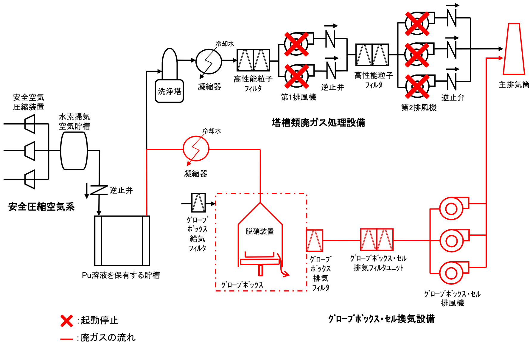
塔槽類廃ガス処理設備及び安全圧縮空気系の停止時の廃ガスの流れ
