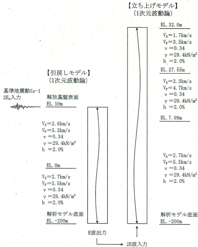
第 4.2-1 図 入力地震動算定の考え方 (1次元地盤モデル)
