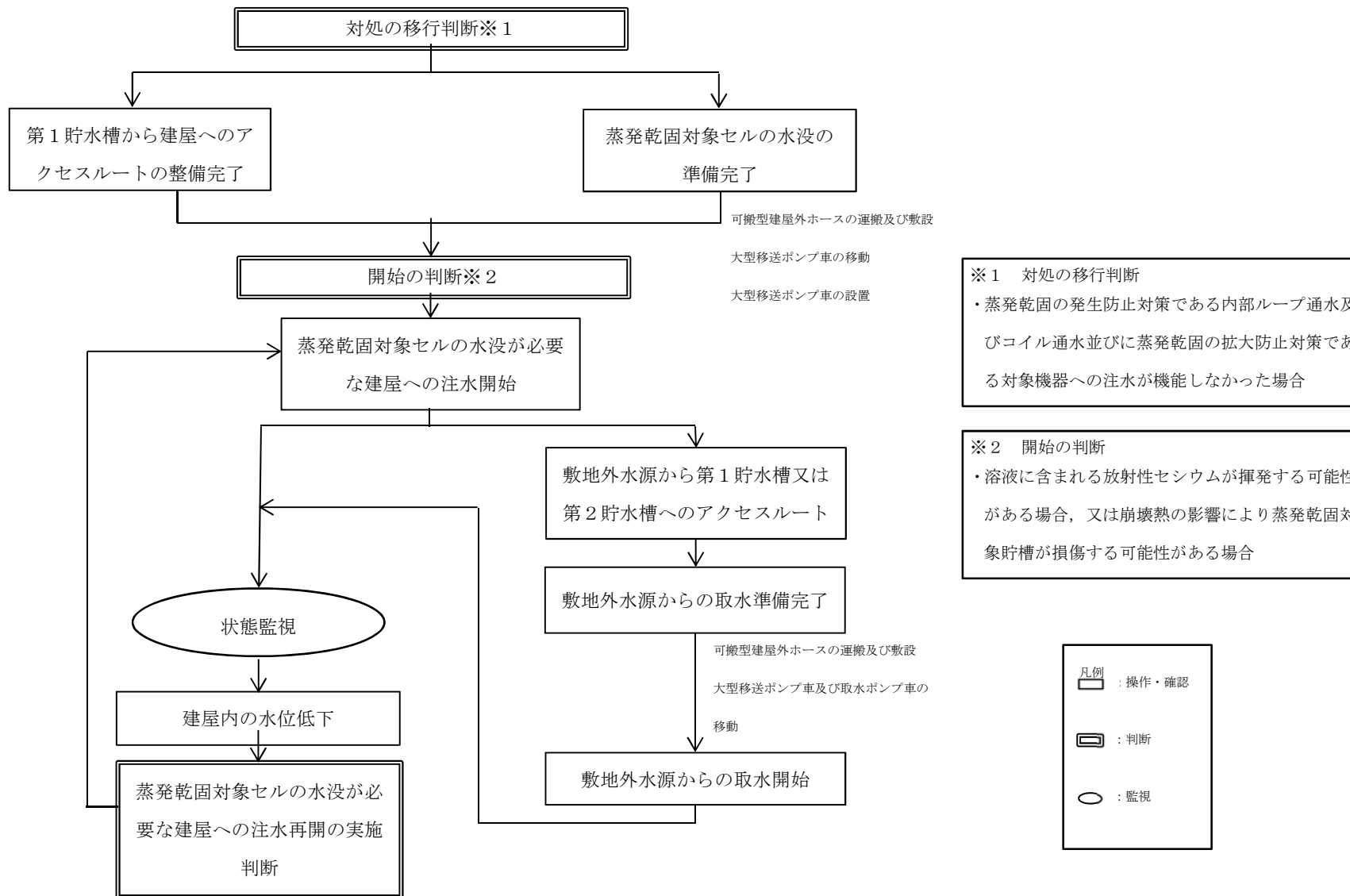
第 5.10.2.1-7 図 「冷却機能の喪失による蒸発乾固対象セルの水没」 の手順の概要
