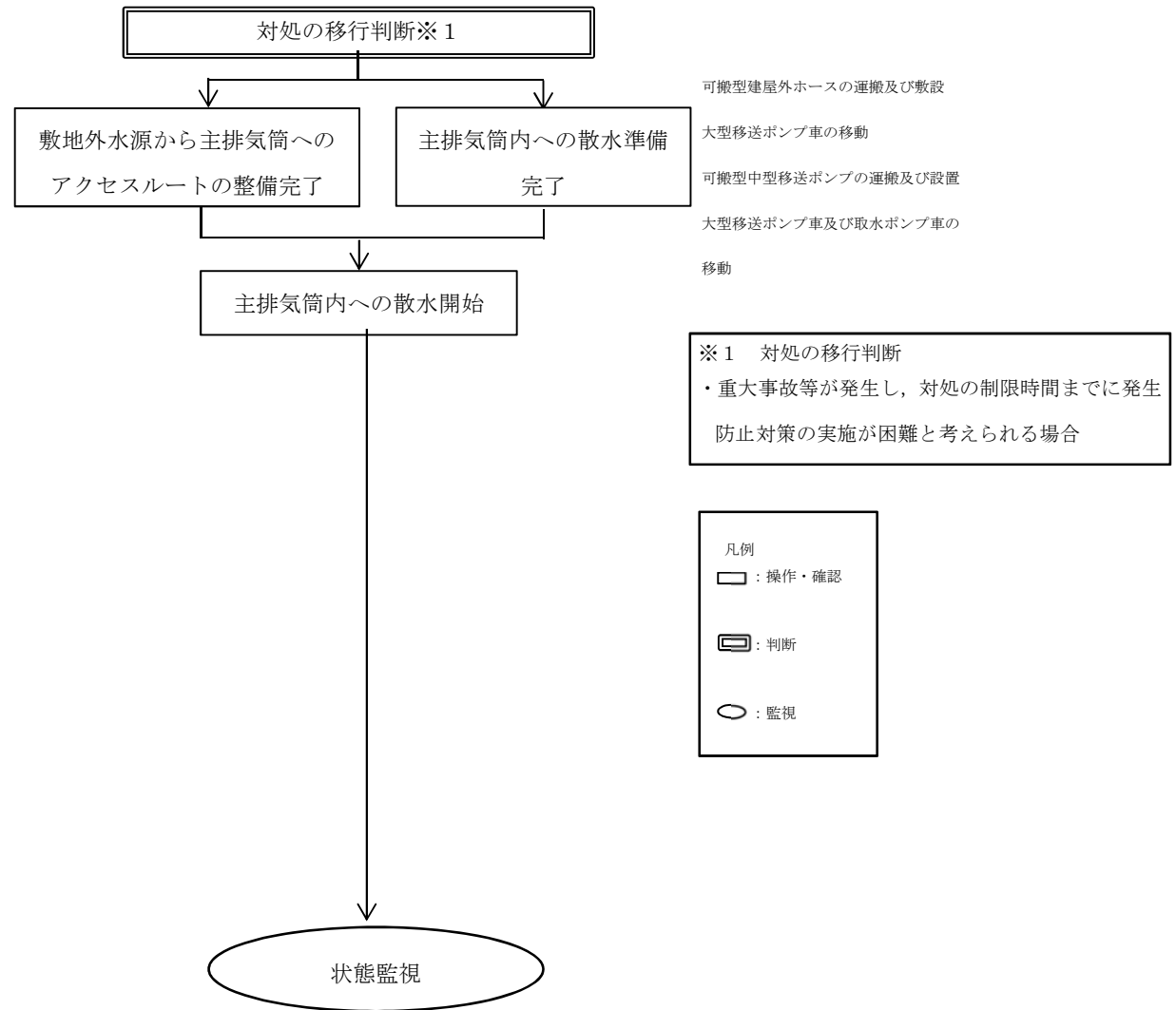
第 5.10.2.1-5 図 「主排気筒内への散水」 の手順の概要
