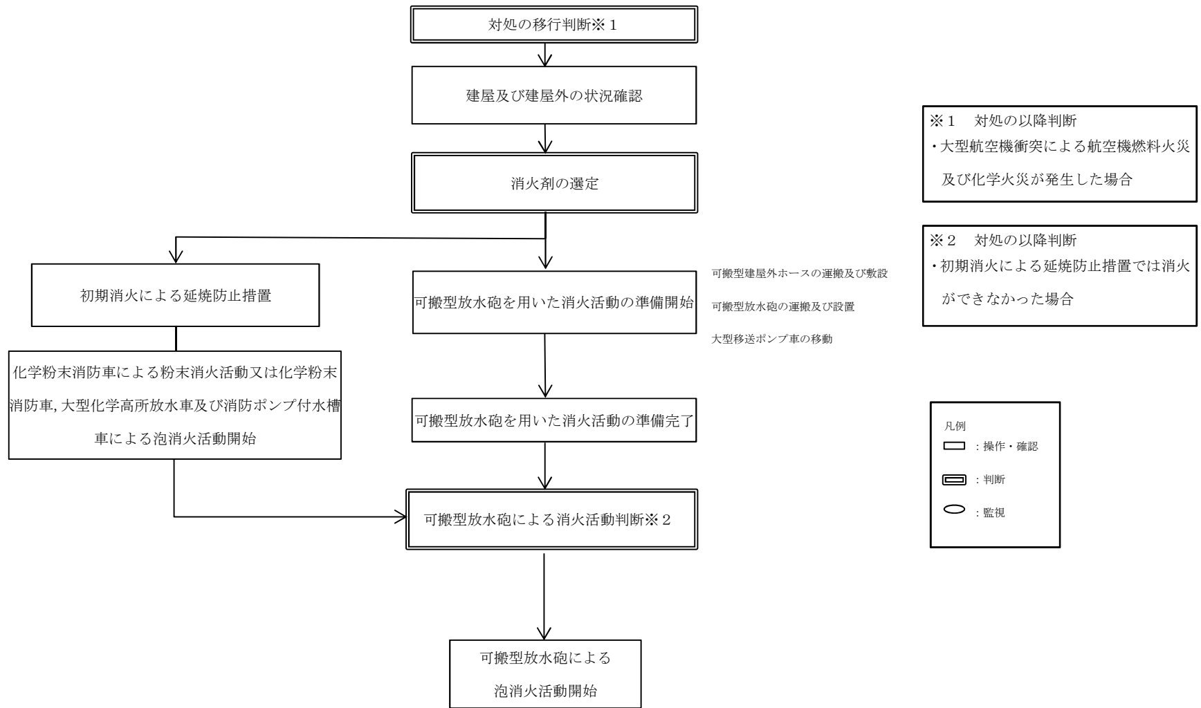
第 5.10.2.1-9 図 「大型航空機衝突による航空機燃料火災及び化学火災の消火活動」 の手順の概要
