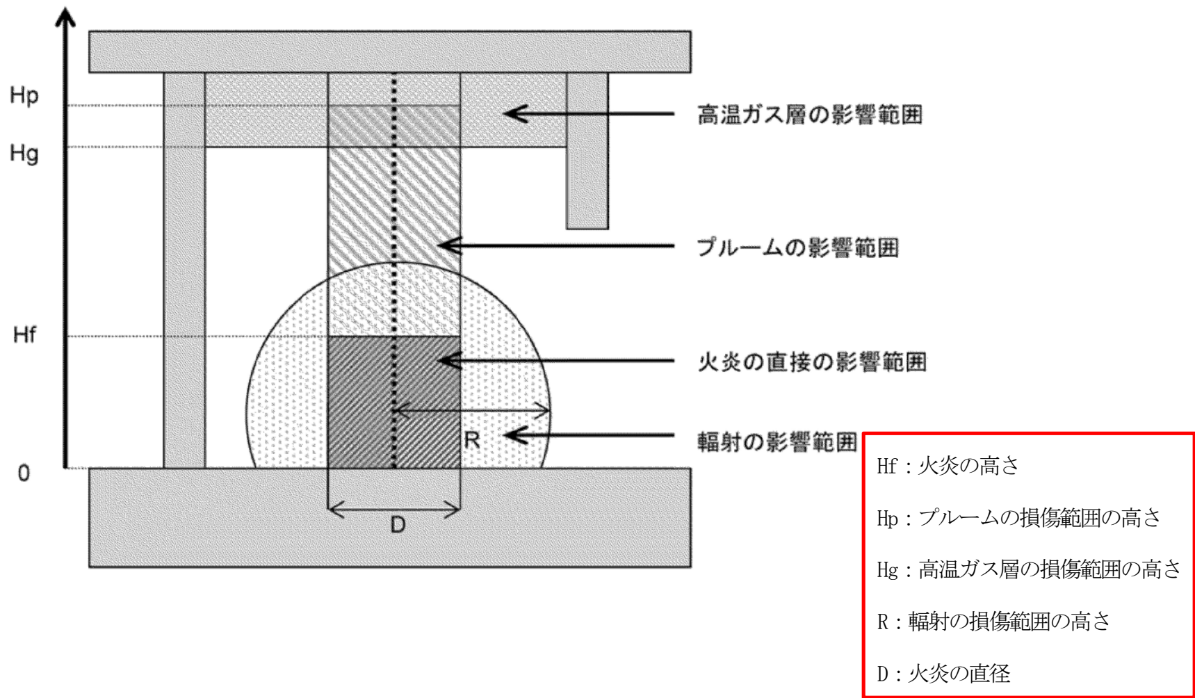
添5第48図 火災影響範囲 (ZOI) 概念図
