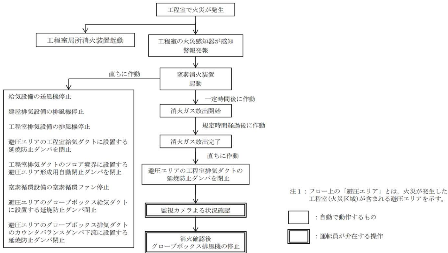
添5第45図 火災区域に設定する工程室の火災発生時の消火対応フロー図
