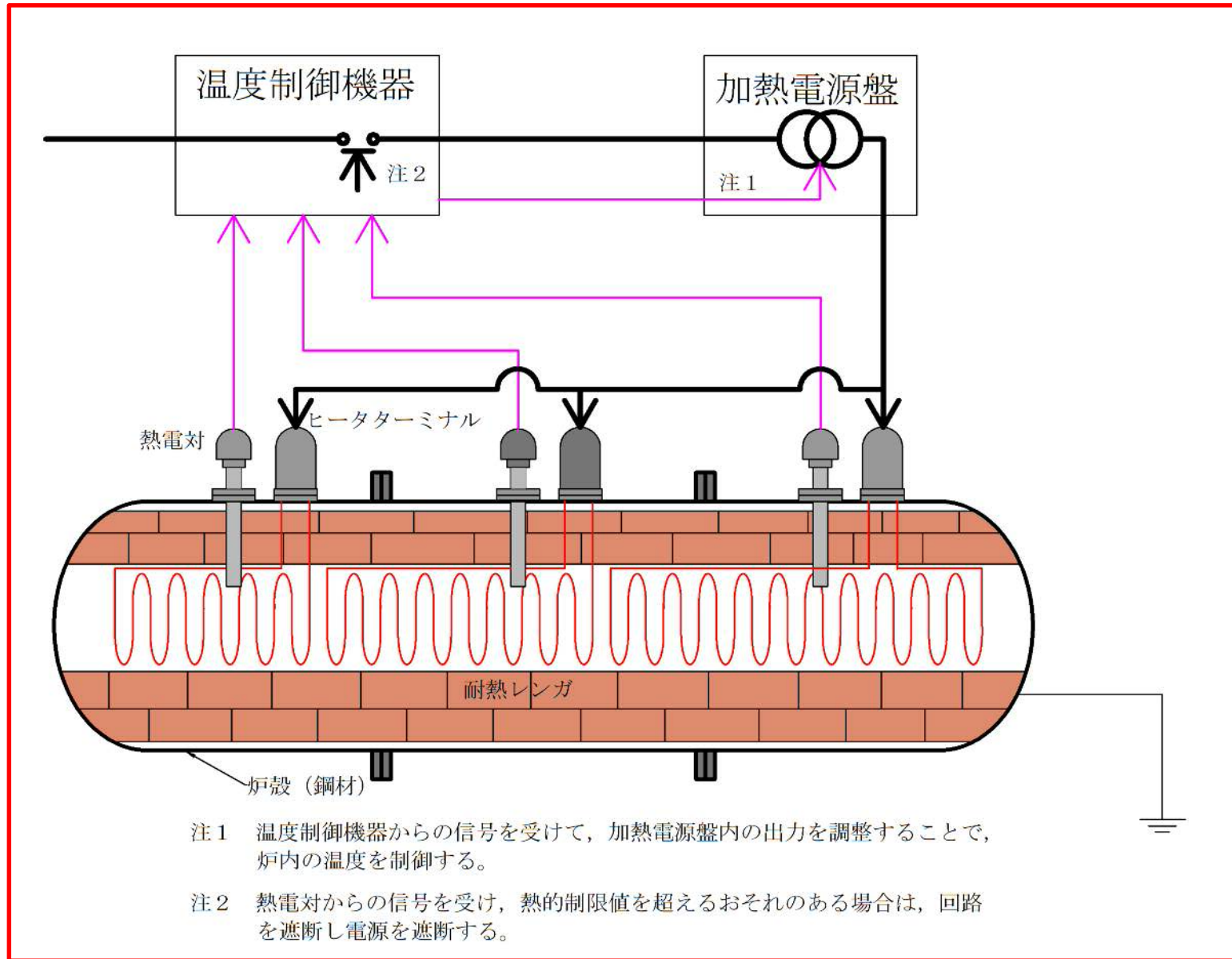
添5第32図 焼結炉の温度制御概念図
