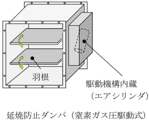
添5 第43 図 延焼防止ダンパの構造の概念図
