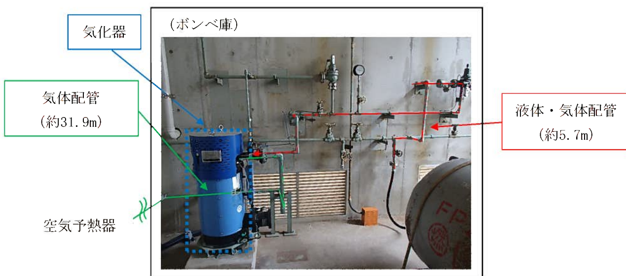
図 雑固体焼却設備のプロパンボンベ気化器周りの現場状況
