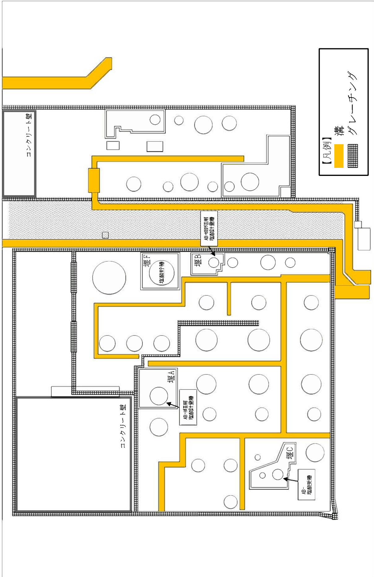
図2 全体図 (1/2号補給水処理装置)
