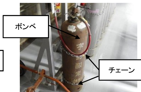
高浜4号炉 タービン建屋 アセチレン (分析用)
