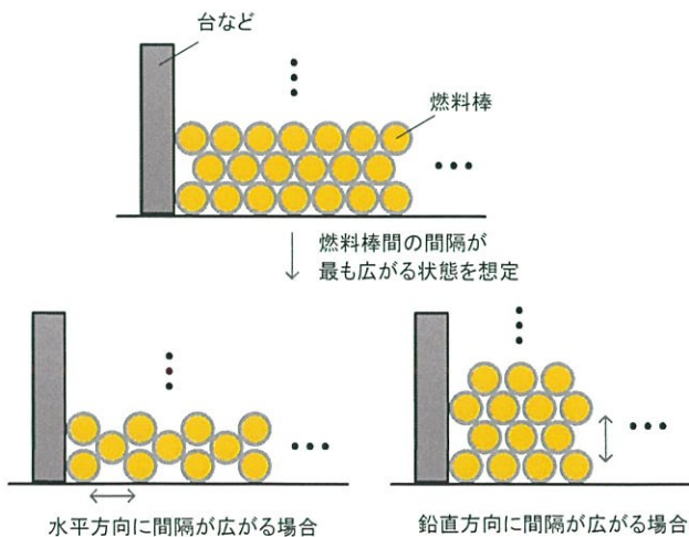
第2図 燃料棒の積み上がり方
