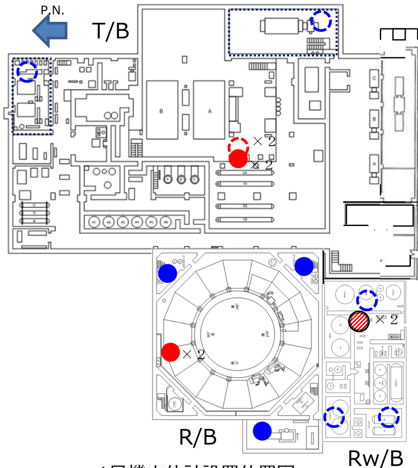
1号機水位計設置位置図
