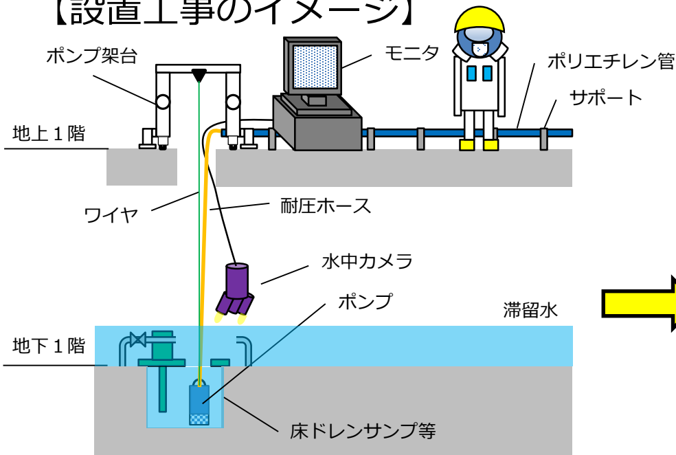
設備設置 【断面図】
