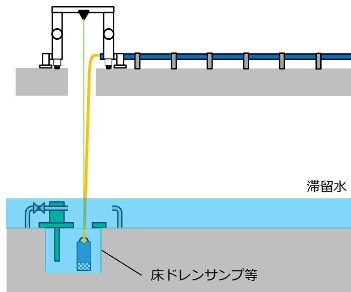
設備設置後 【断面図】
