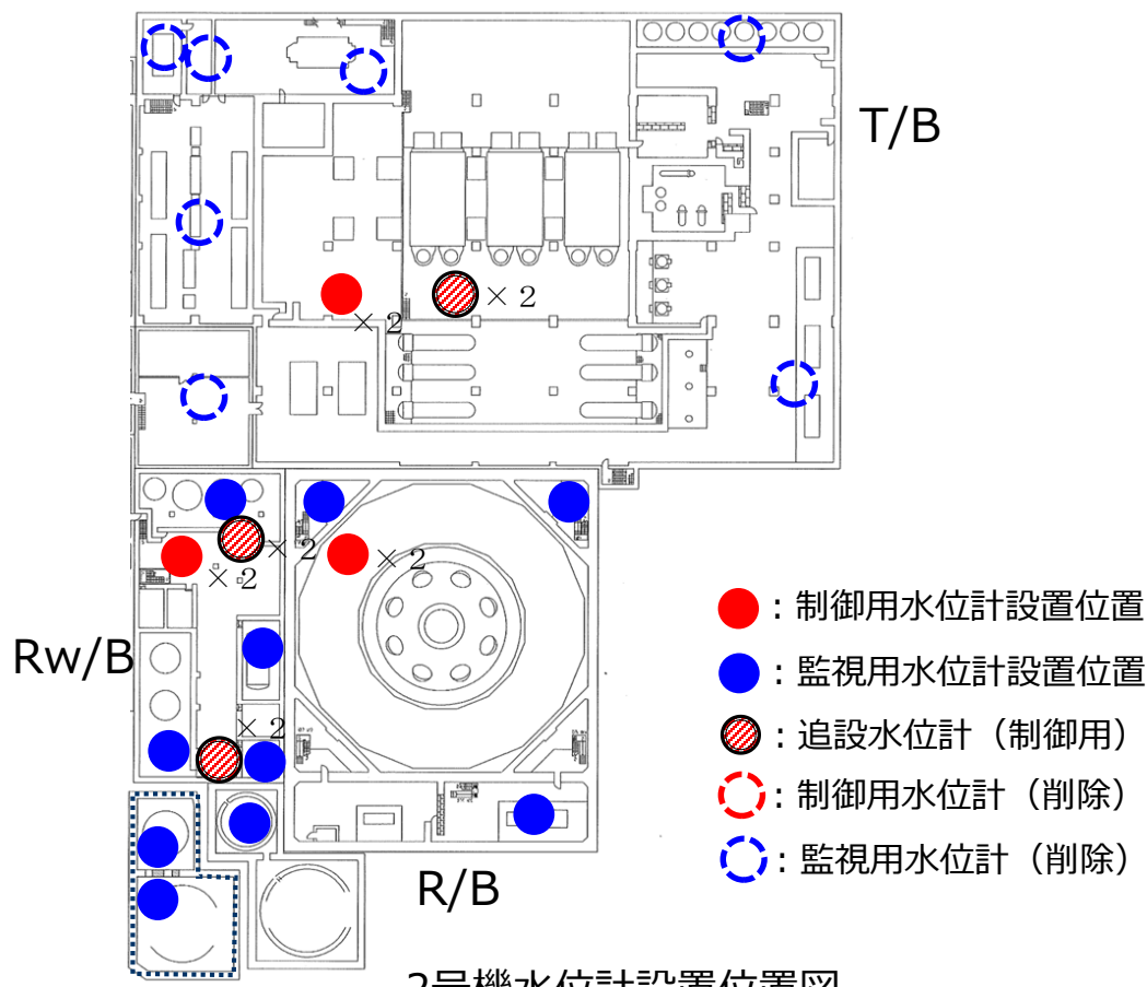
2号機水位計設置位置図
