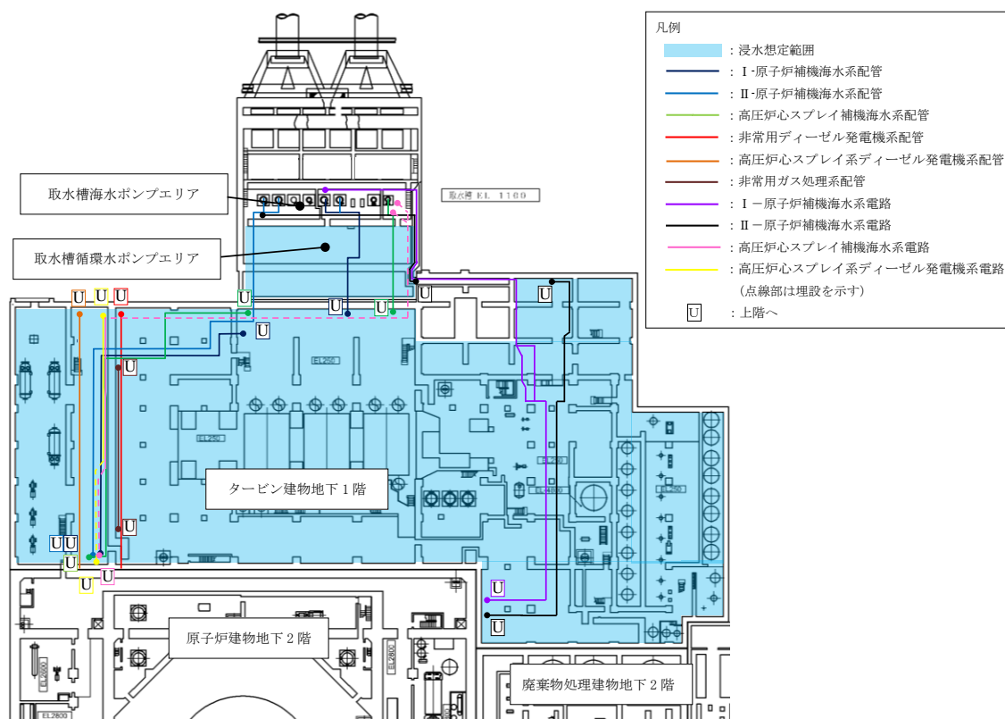
図 9-9 防護対象設備配置図
