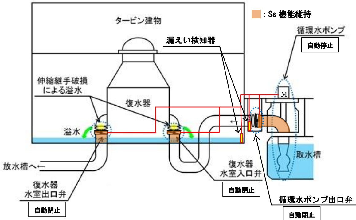
図 9-2 循環水ポンプ停止及び循環水系弁閉止 インターロック設置概要図
