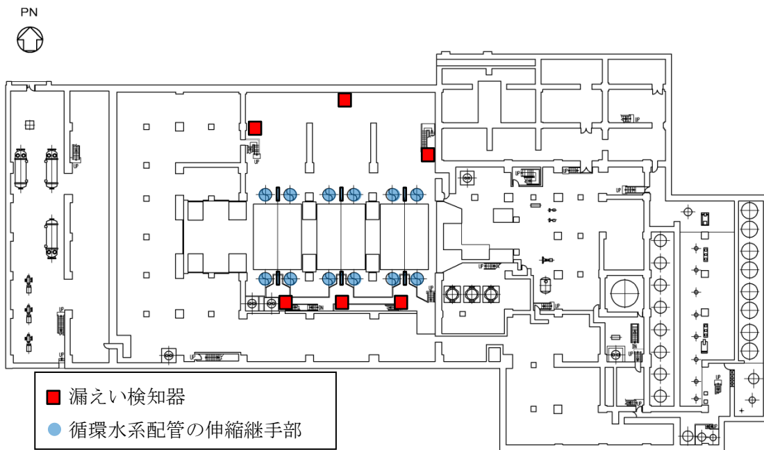
図 9-4 漏えい検知器設置箇所 (タービン建物地下1階)
