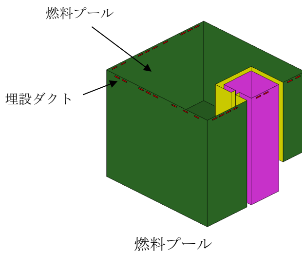
図 8-5 解析モデル図
