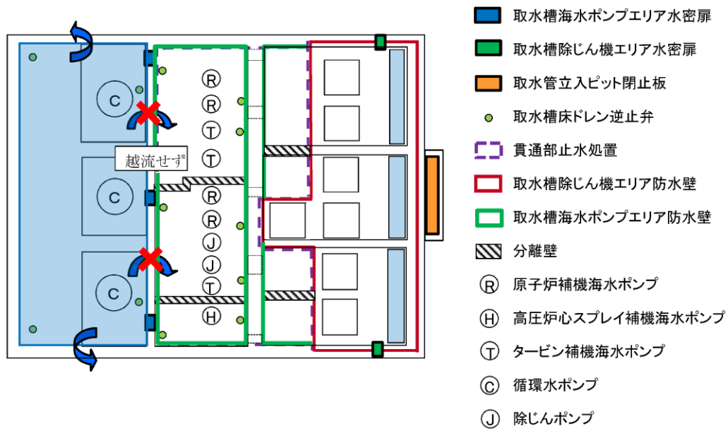
図 9-10 海水ポンプエリア平面図（循環水系配管破損時）
