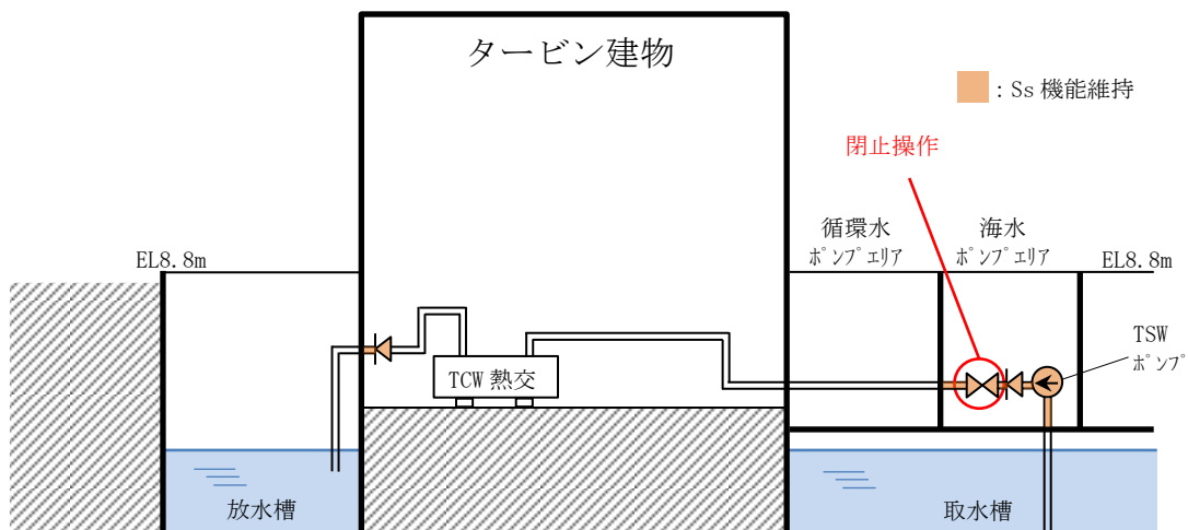
図 9-8 タービン補機海水系概要図
