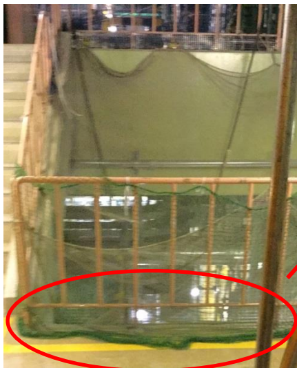
図3 想定した溢水経路に影響を与える可能性のある設備の確認例 (原子炉建物中2階)
