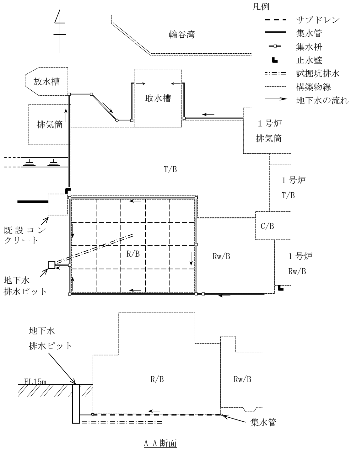
図10-4 地下水排水設備の概要
