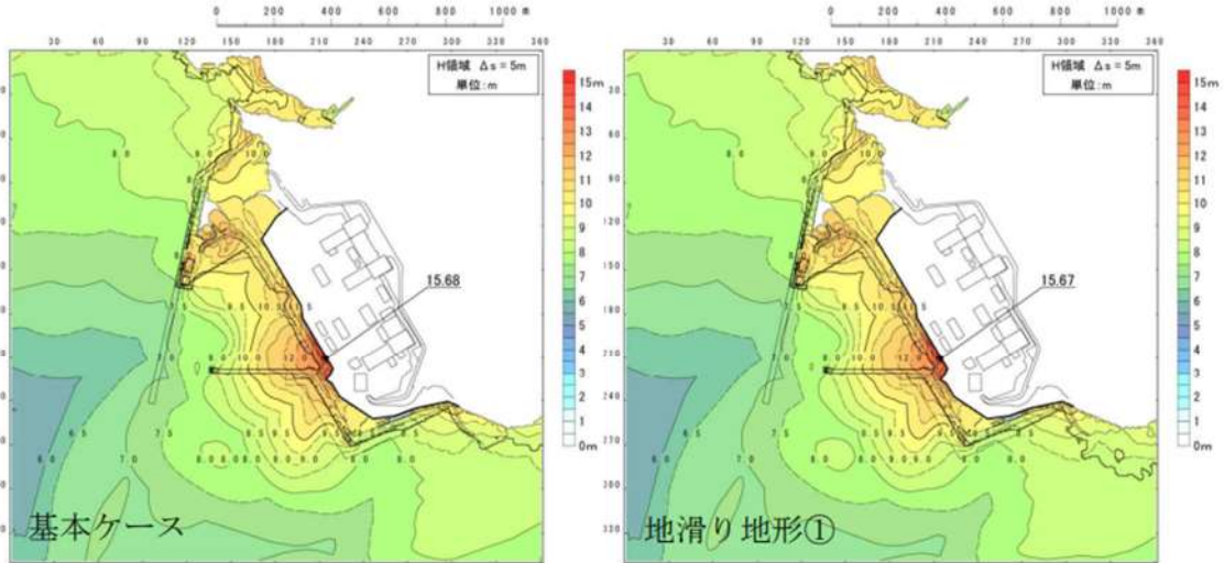
図 2.1. b. c-1 (23) 地滑り地形①の斜面崩壊の有無による最大水位上昇量分布の比較（基準津波（波源F，北防波堤損傷））
