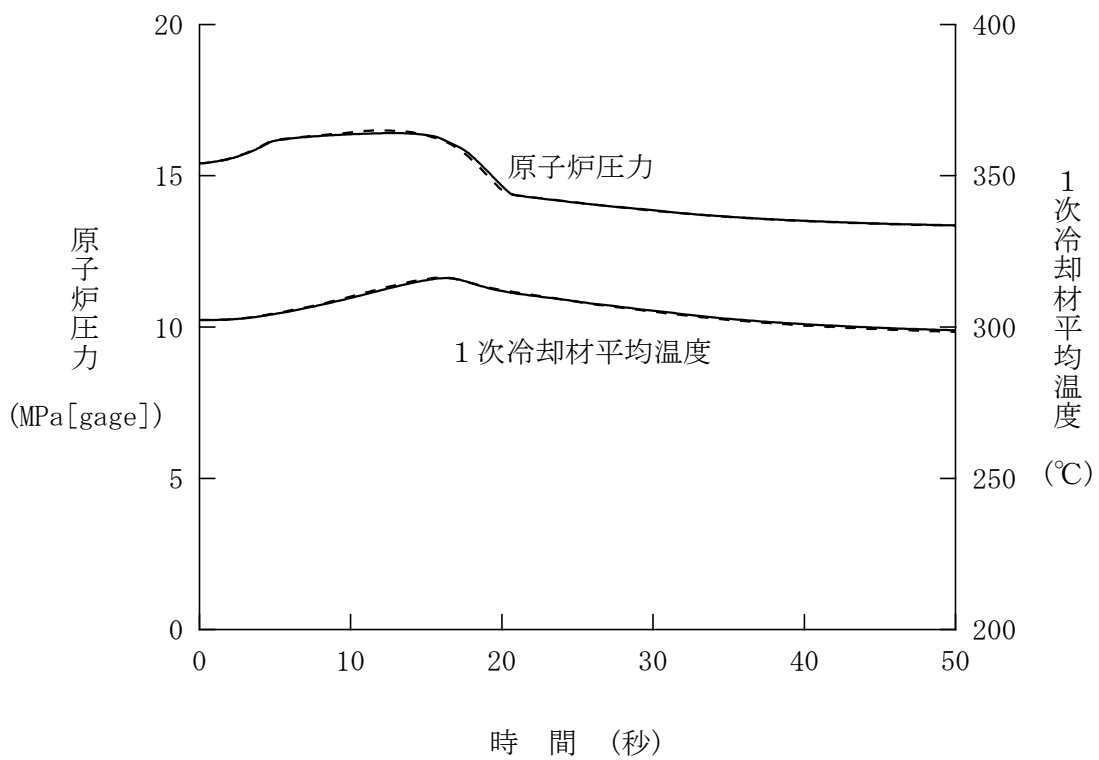
図 2 蒸気発生器取替え前後の解析の比較 (負荷の喪失-加圧器圧力制御系作動)
