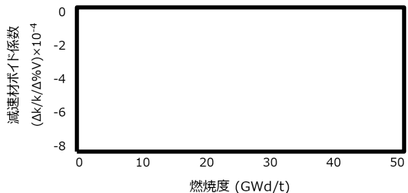
減速材ポイド係数 (9x9燃料 (A型) 取替燃料) への影響例
