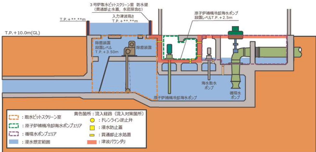
第 1.5. ● 図 3号炉取水系統 浸水対策配置図 (A-A 断面図)
