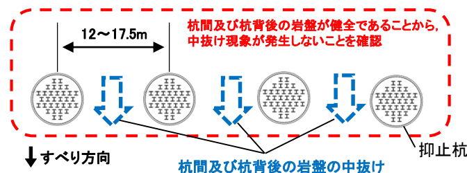
図6 概念図
