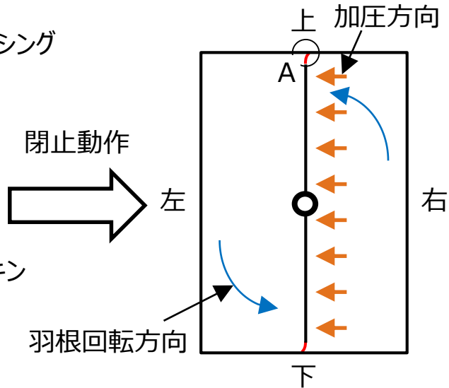
ダンパ閉止時断面概要
