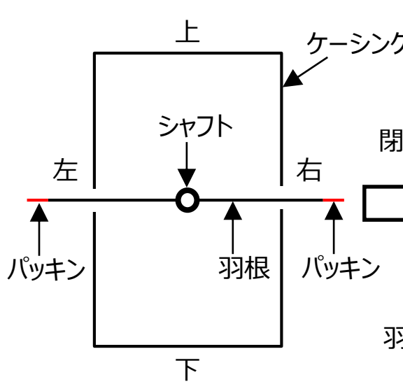
ダンパ開放時断面概要 左：建物屋内側 右：建物屋外側 (加圧側)
