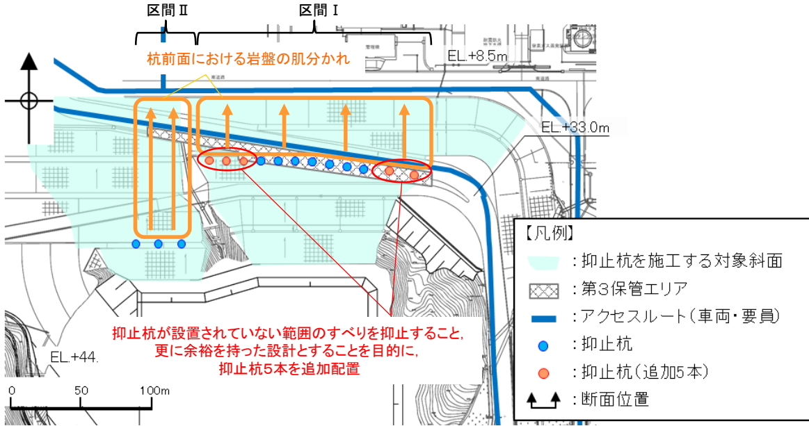
図3 平面図
