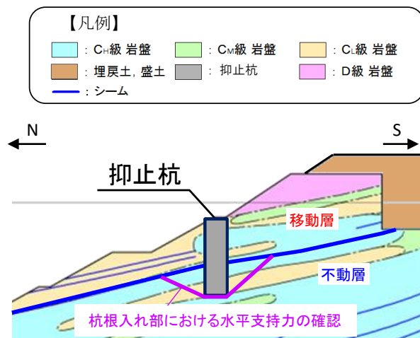
図5 断面図
