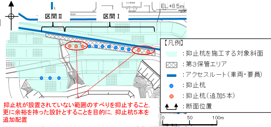
図7 平面図
