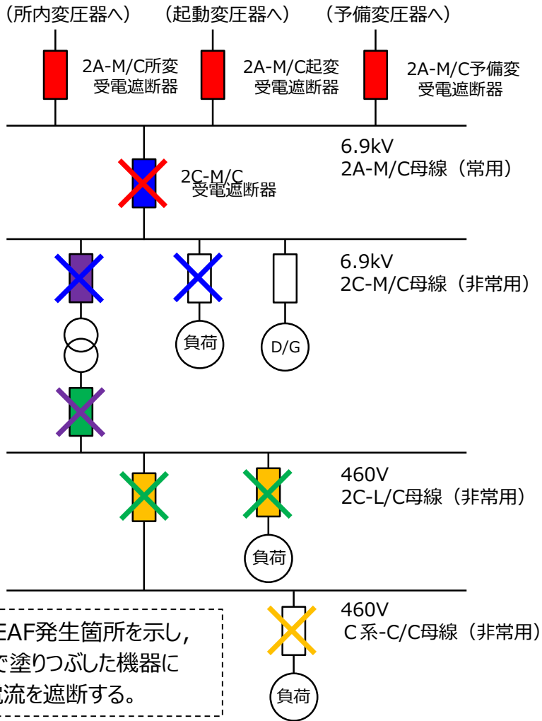
図4 系統給電
