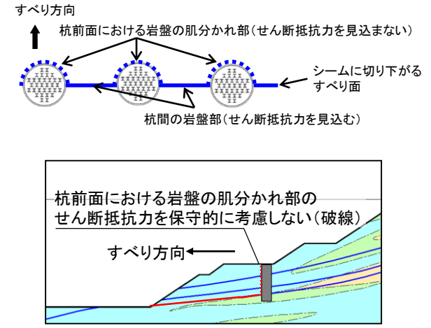
図4 杭前面と岩盤の肌分かれの考慮（イメージ図）
