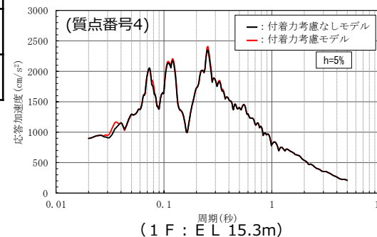
図3 原子炉建物の床応答スペクトル(NS方向, h=5%)の比較
