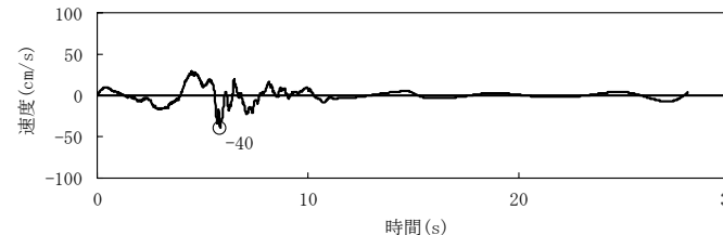
実観測記録の位相による時刻歴波形(水平方向)
