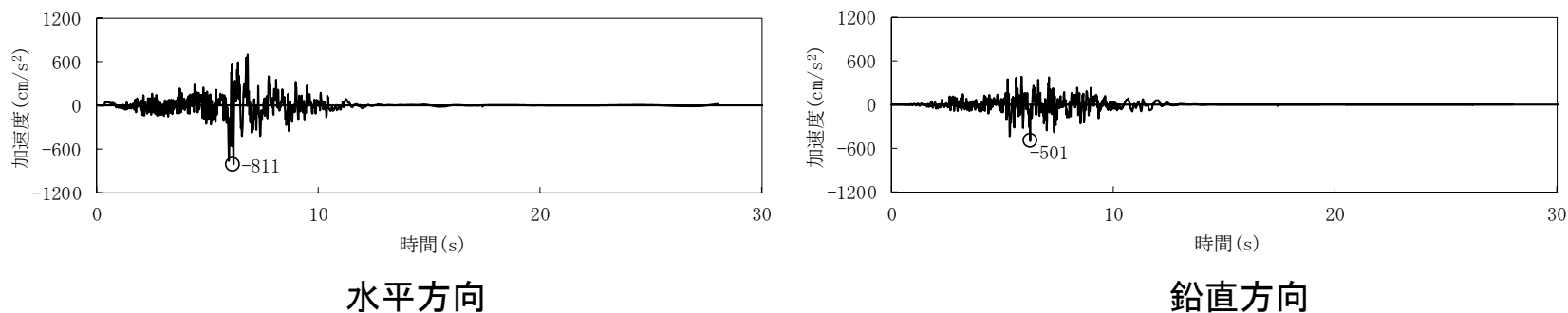
解放基盤表面における加速度時刻歴波形
