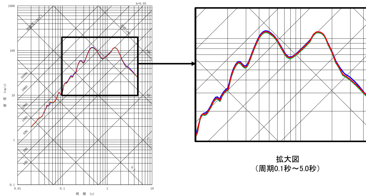
水平方向 擬似速度応答スペクトル
