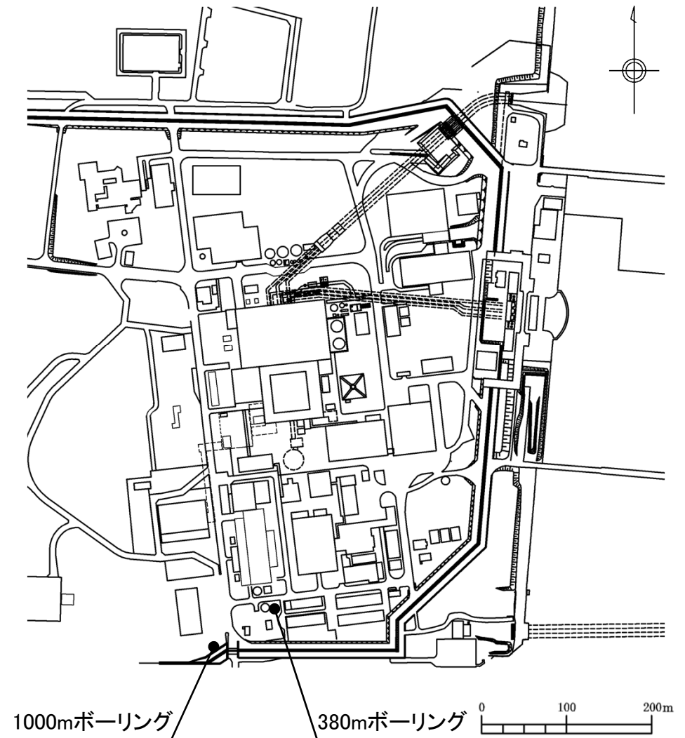
地盤モデルの検討に用いた ボーリング位置(平面)
