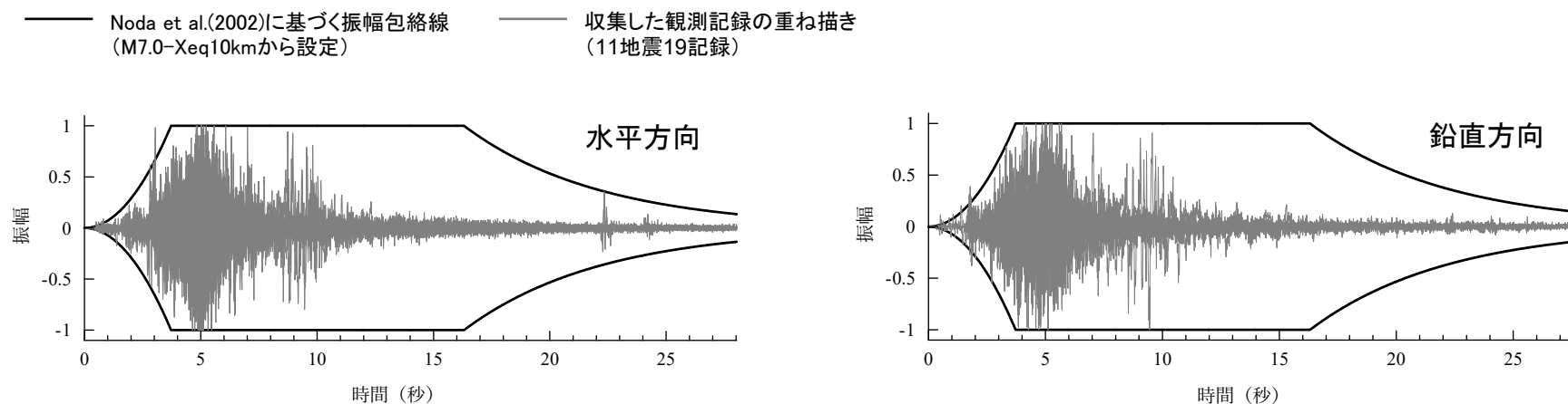
収集した観測記録(11地震19記録)の加速度時刻歴波形の重ね描き(振幅を基準化)※
