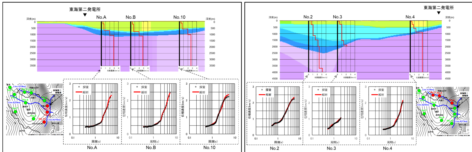
屈折法地震探査のLine-A測線付近で実施した微動アレイ探査結果
