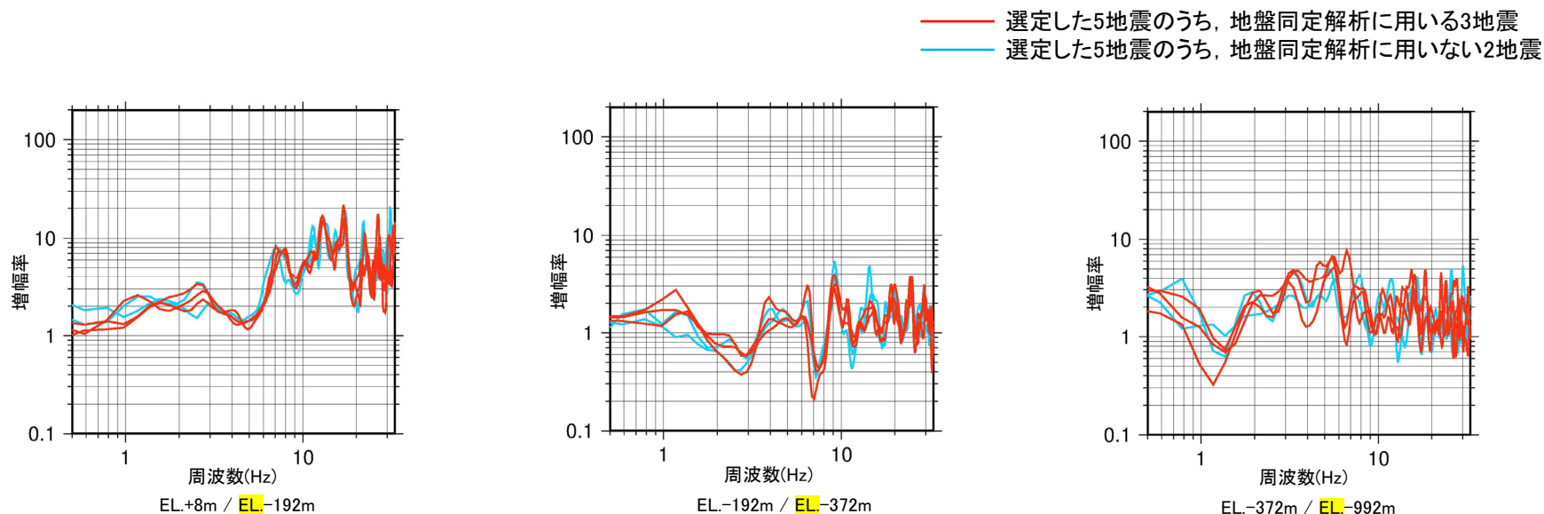
選定した5地震の伝達関数(UD方向)
