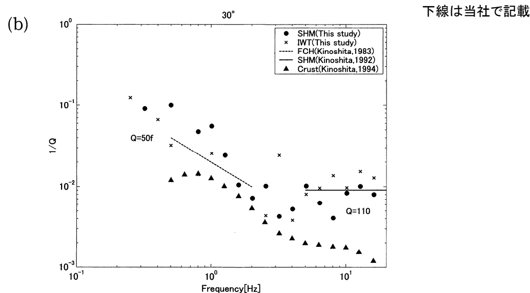
(b) フーリエ振幅スペクトルを1/3オクターブ帯域幅で平滑化した場合
