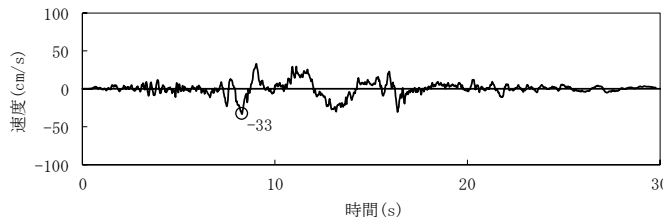
乱数位相による時刻歴波形(水平方向)
