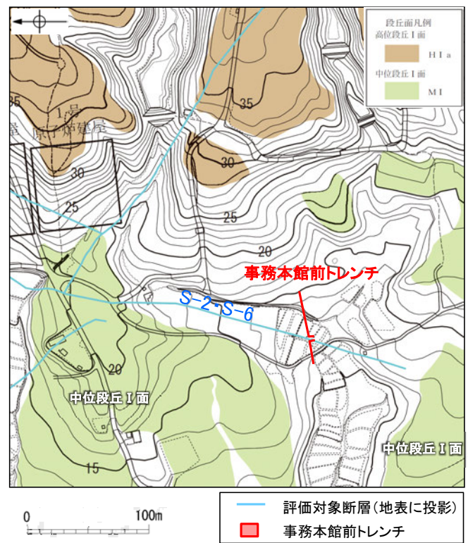
位置図
