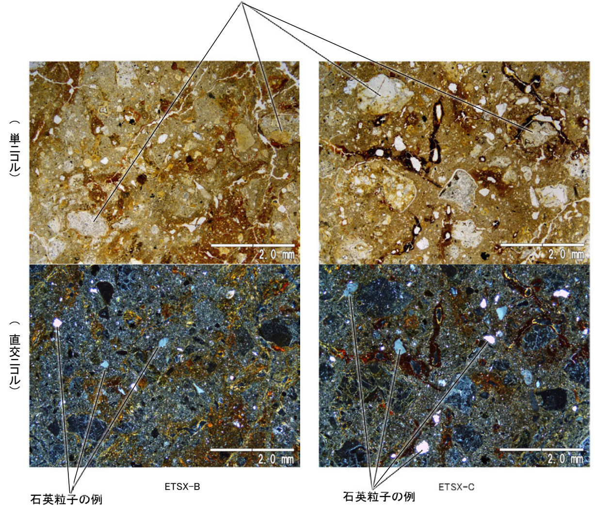
薄片写真
