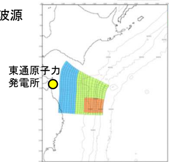
波源モデル
