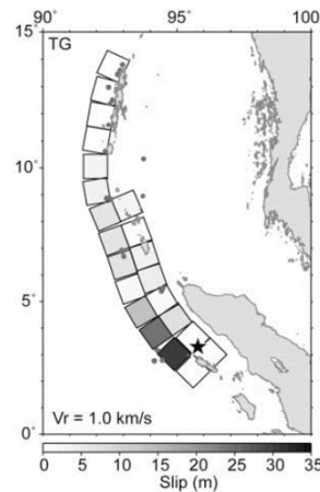
2004年スマトラ～アンダマン地震 (Fujii and Satake (2007))
