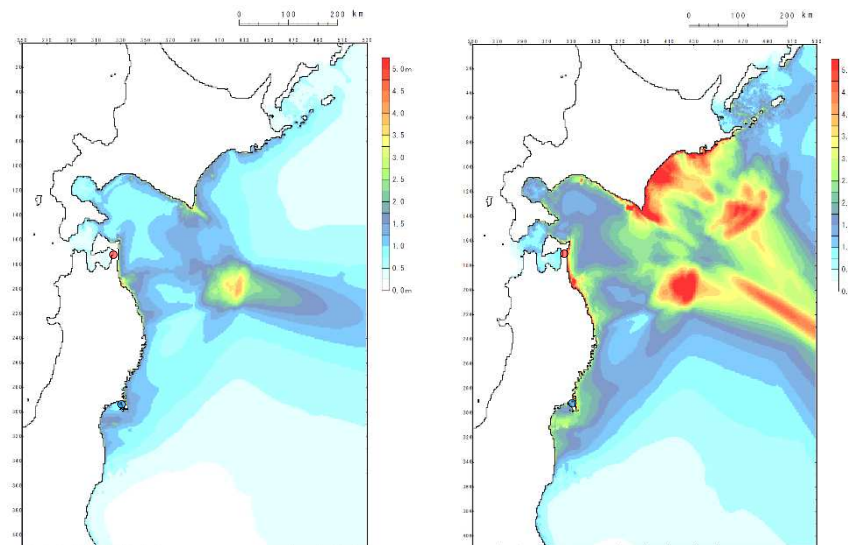
十勝沖・根室沖から岩手県沖北部
