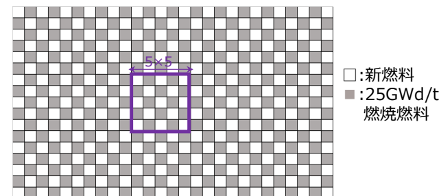
図1 燃料配置、燃焼度条件
