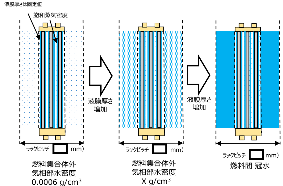
パラスタ④-2のイメージ
