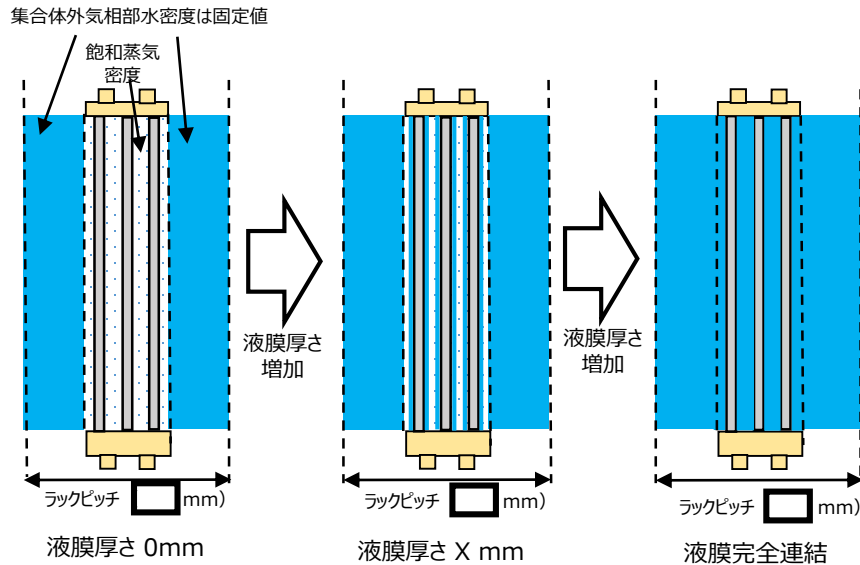
パラスタ④-1のイメージ
