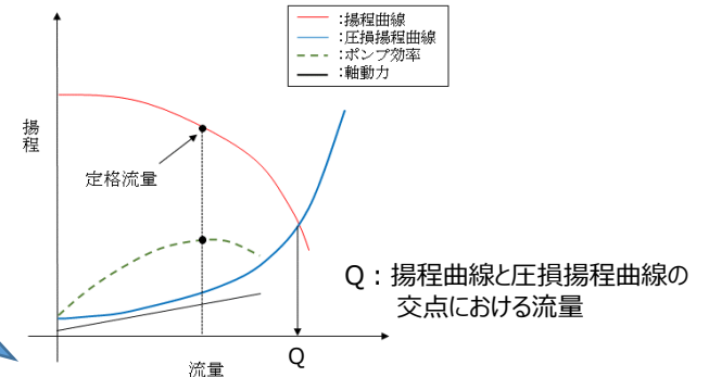
図 ポンプ揚程曲線を用いた流量の算出方法概略
