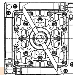
参考図 内挿物（プラグングデバイス）が挿入された燃料集合体の上面
