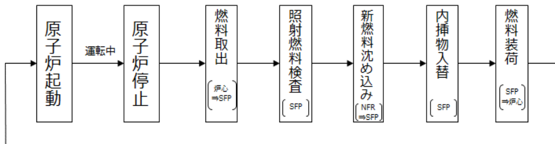
図 PWRでの燃料取替に係る工程
