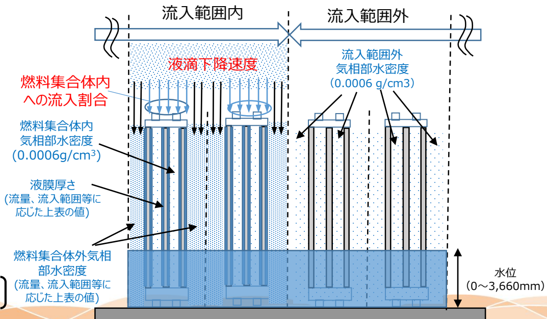
図 臨界計算コードへのインプットとなる水分条件 概要
