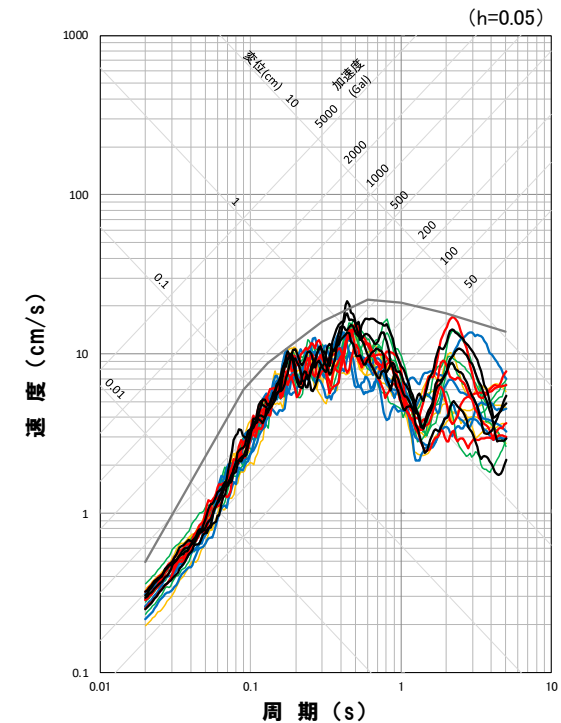
応答スペクトル図(UD方向)
