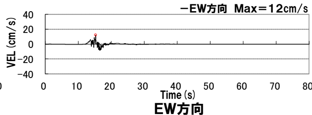
積丹半島北西沖の断層による地震(走向40° ケース, 基本震源モデル, 破壊開始点4)
