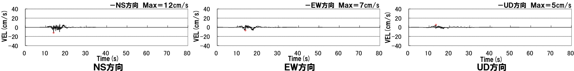
積丹半島北西沖の断層による地震(走向20° ケース, 基本震源モデル, 破壊開始点4)
