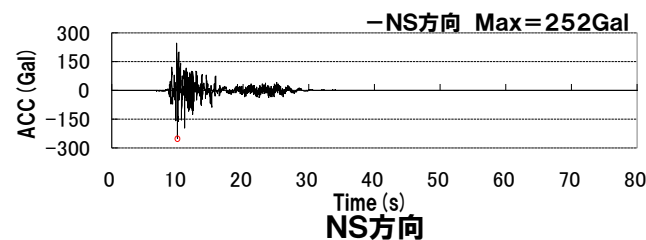
尻別川断層による地震(不確かさ考慮モデル(応力降下量), 破壊開始点1)
