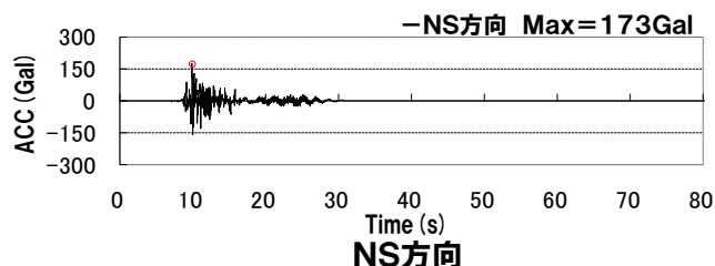
尻別川断層による地震(基本震源モデル, 破壊開始点1)
