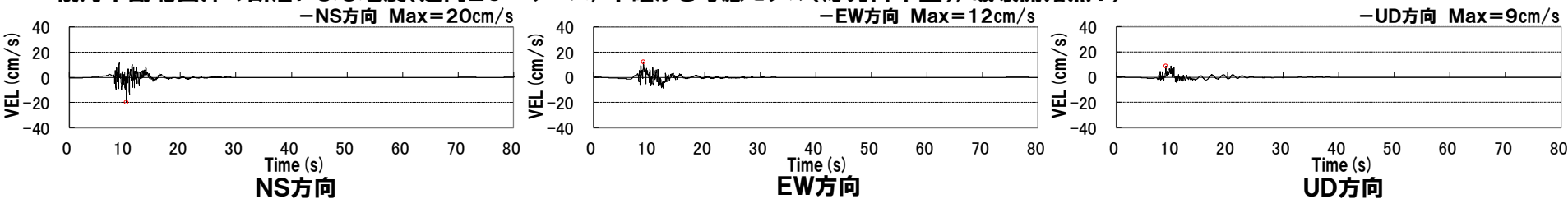
積丹半島北西沖の断層による地震(走向20° ケース, 不確かさ考慮モデル(応力降下量), 破壊開始点2)
