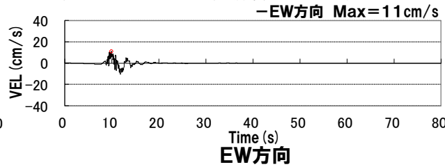
積丹半島北西沖の断層による地震(走向40° ケース, 基本震源モデル, 破壊開始点2)
