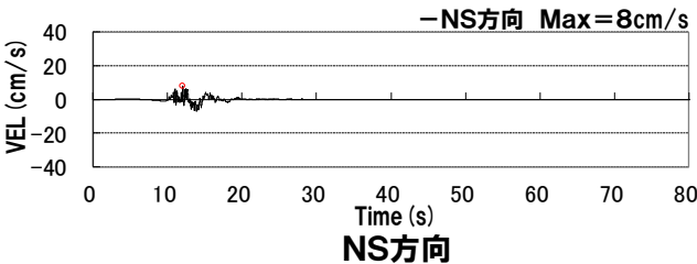
積丹半島北西沖の断層による地震(走向40° ケース, 基本震源モデル, 破壊開始点3)
