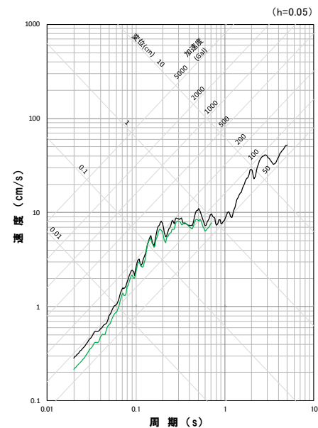
応答スペクトル図(UD方向)
