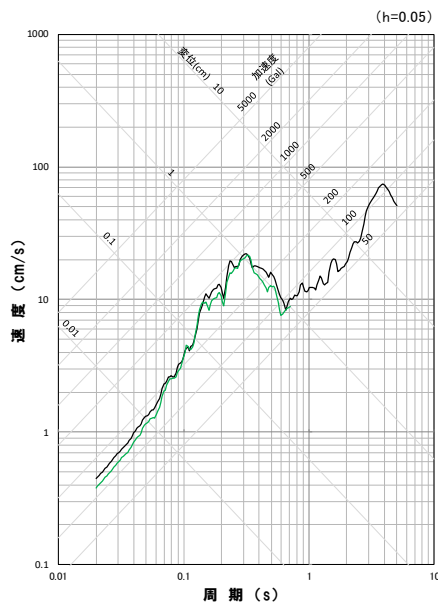
応答スペクトル図(NS方向)
