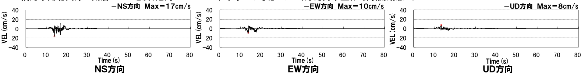
積丹半島北西沖の断層による地震(走向20° ケース, 不確かさ考慮モデル(応力降下量), 破壊開始点4)
