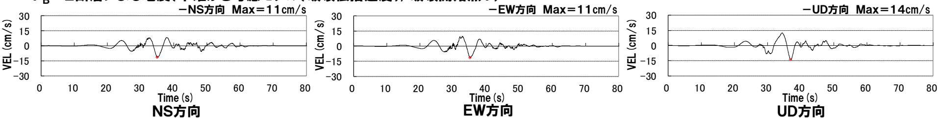
F_B-2 断層による地震(不確かさ考慮モデル(破壊伝播速度), 破壊開始点2)
