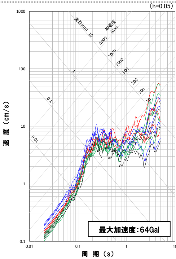
応答スペクトル図(EW方向)
