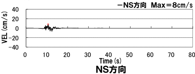
積丹半島北西沖の断層による地震(走向40° ケース, 基本震源モデル, 破壊開始点2)
