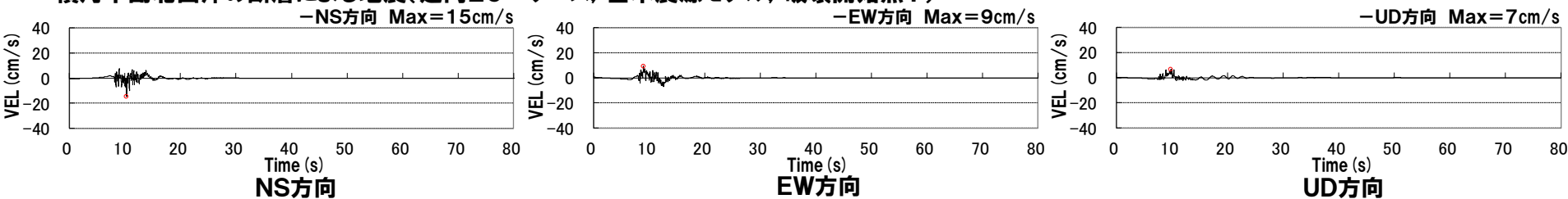
積丹半島北西沖の断層による地震(走向20° ケース, 基本震源モデル, 破壊開始点2)
