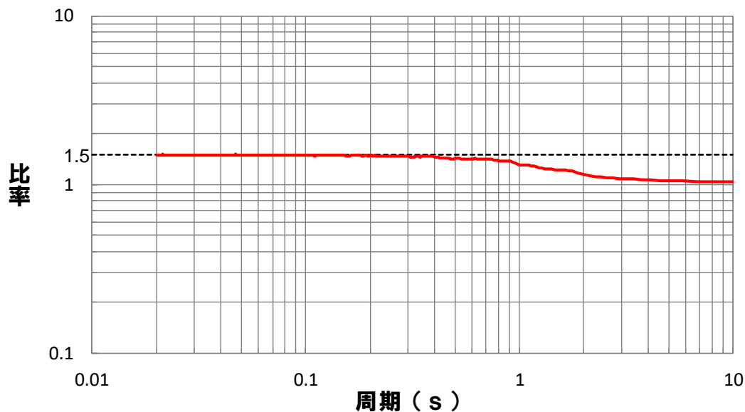
尻別川断層による地震 フーリエスペクトル比 (不確かさ考慮モデル(応力降下量)/基本震源モデル)
