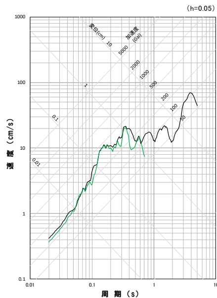
応答スペクトル図(EW方向)
