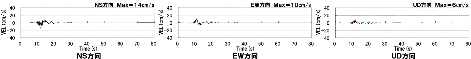
積丹半島北西沖の断層による地震(走向20° ケース, 基本震源モデル, 破壊開始点3)
