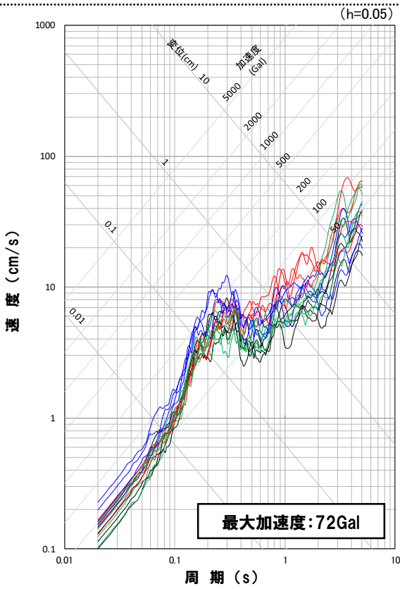
応答スペクトル図(NS方向)
