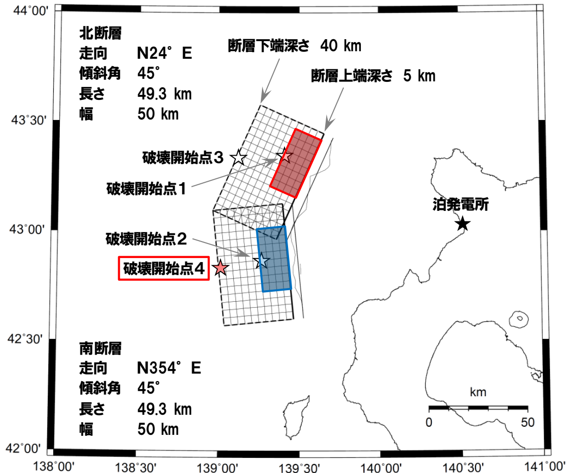
基本震源モデル
