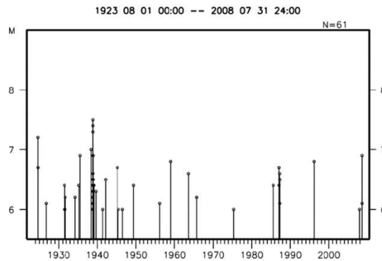
上図:震央分布図(1923年~2008年, M \geq 6.0)
