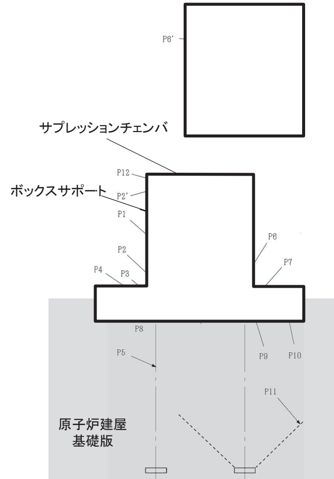
ボックスサポートの応力評価点
