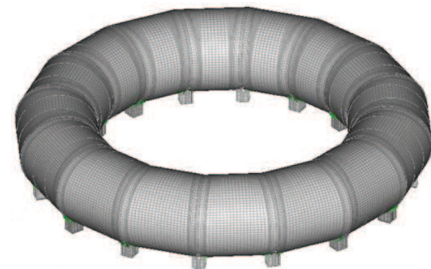
適用性確認用解析モデル(3次元シェルモデル)
