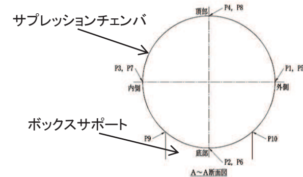
サプレッションチェンバ本体の応力評価点
