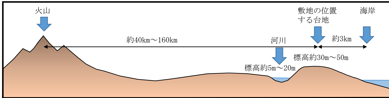
敷地周辺の河川及び海岸等との位置関係図
