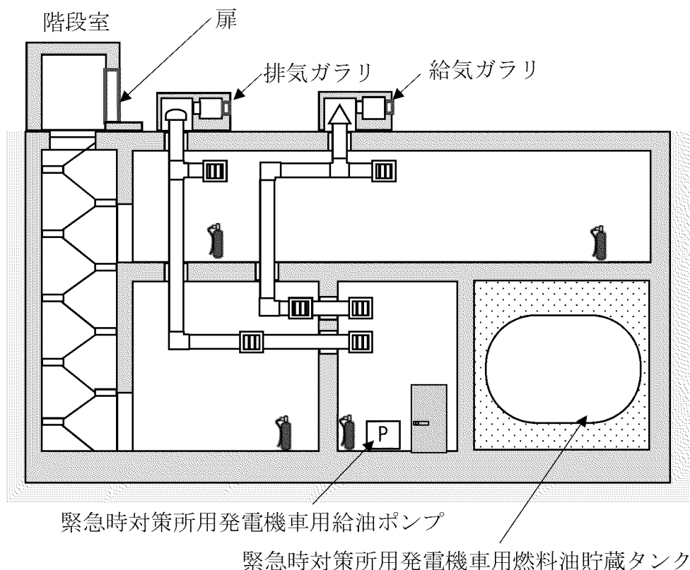
図 6-2 緊急時対策棟屋外地下エリア 換気系統概要図
