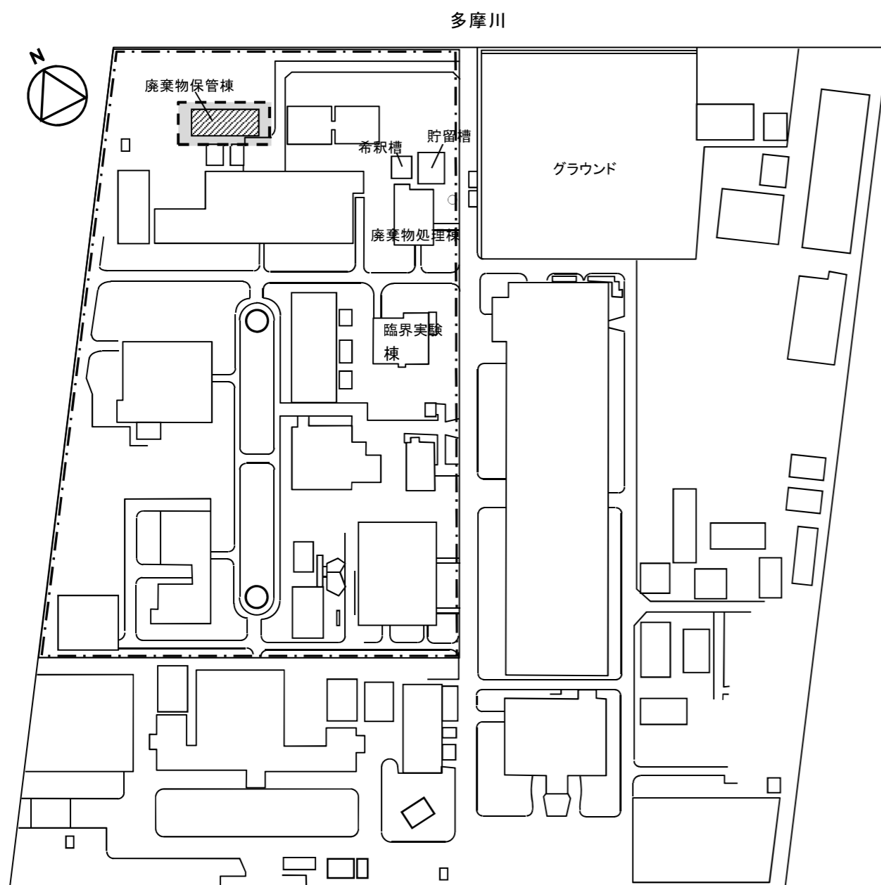
図7-5 廃棄物保管棟の建設エリア
