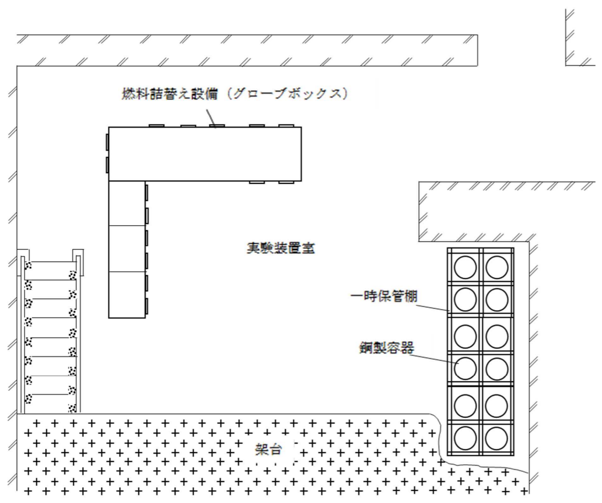
図7-1 燃料詰替え設備の配置概要
