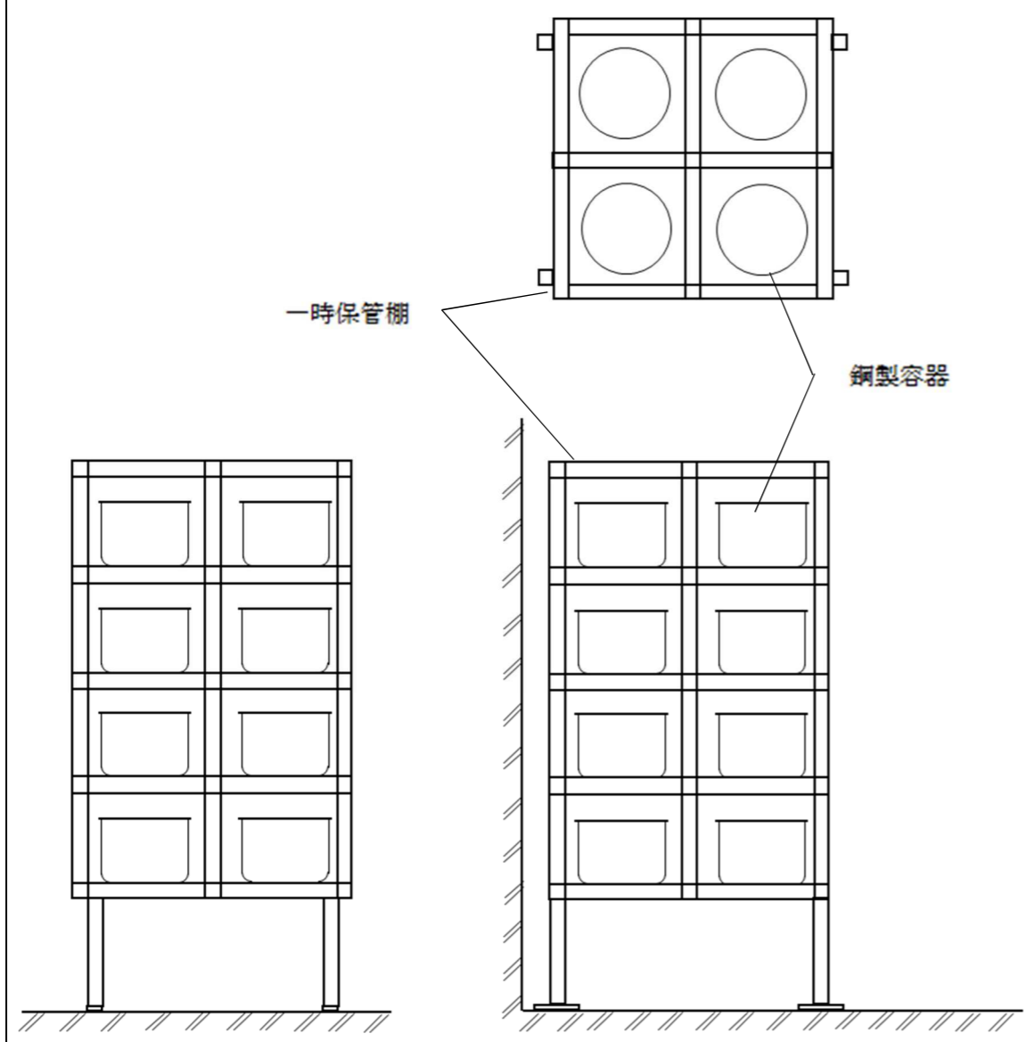
図7-3 鋼製容器の一時保管棚
