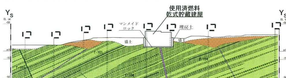
Y_S-Y_S' 断面
