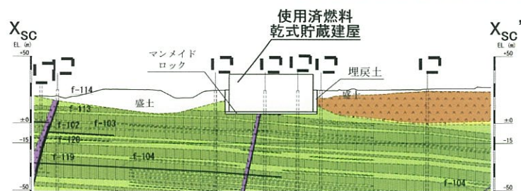
X_{SC}-X_{SC}' 断面
