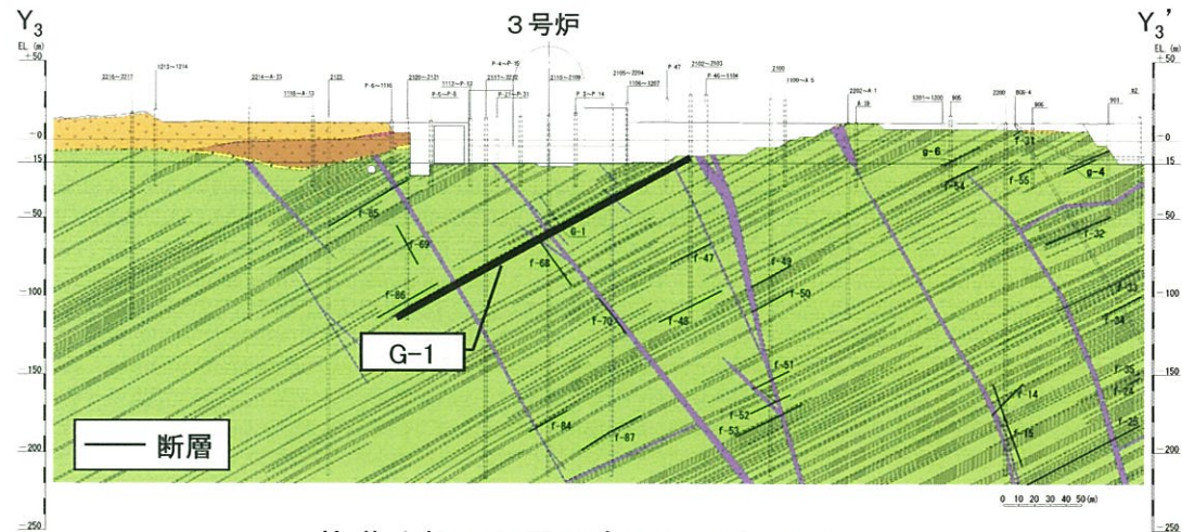
基礎地盤の断層分布 (Y 3 -Y 3 ' 断面)
