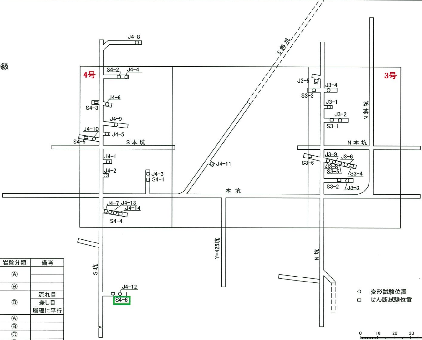
岩盤せん断試験実施位置(玢岩◎級)
