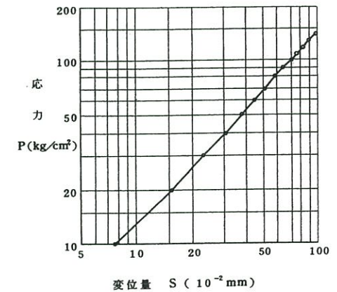
J4-9試験結果 (頁岩③級)
