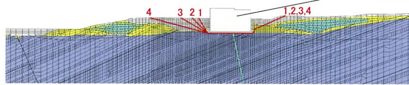
No.3) 断層・シームのすべり (Case1~4)
