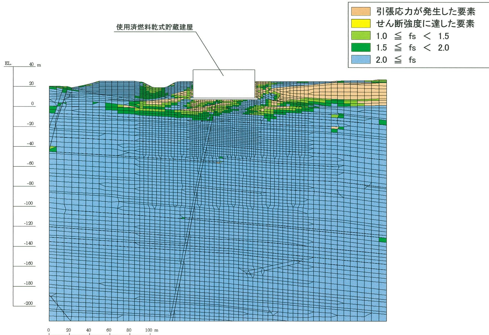
最小すべり安全率発生時刻の局所安全係数図( X_{SC}-X_{SC}' 断面、Ss-1、5.03秒)(応力再配分前)
