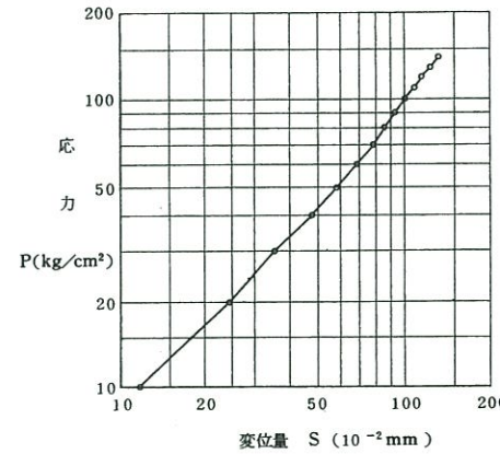
J3-4試験結果 (砂岩③級)
