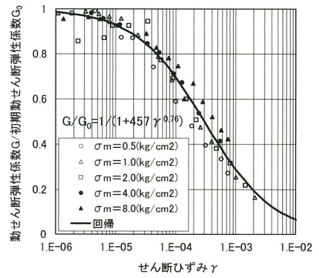
動的変形特性( G_d/G_0 \sim \gamma )
