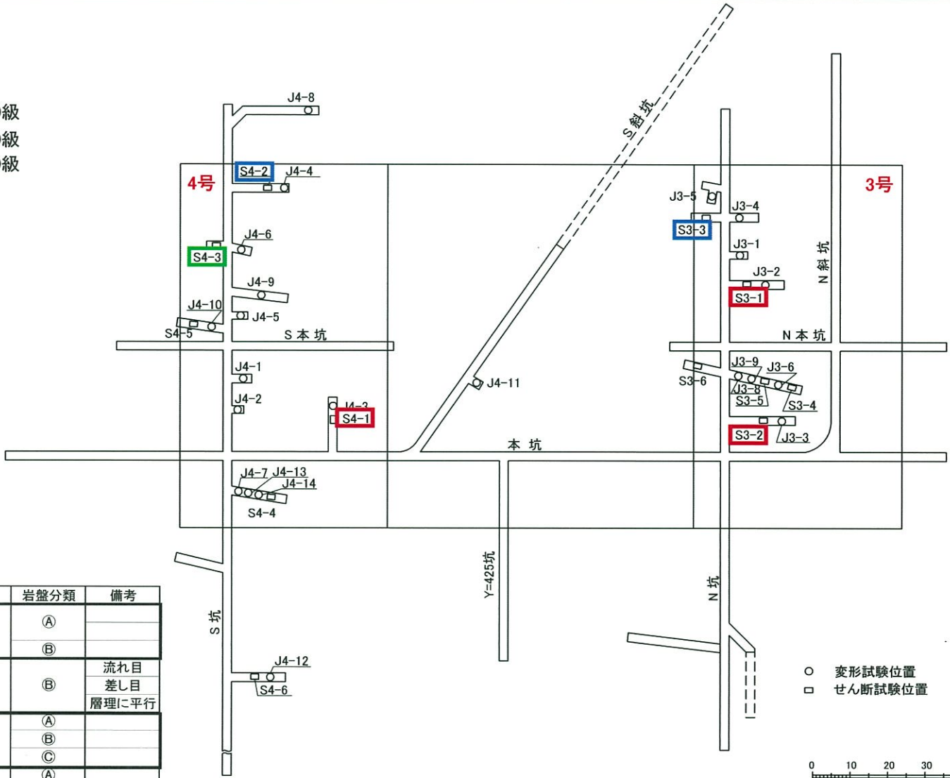
岩盤せん断試験実施位置(砂岩)
