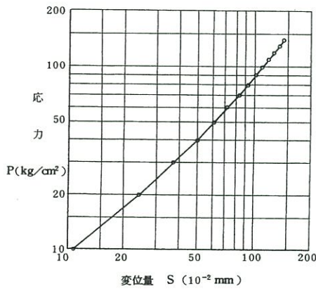
J4-4試験結果 (砂岩③級)
