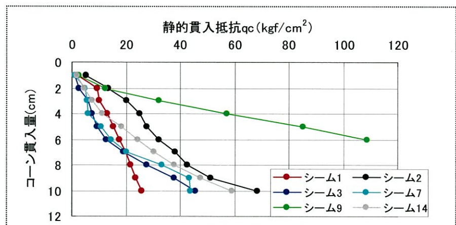
コーン貫入試験結果
