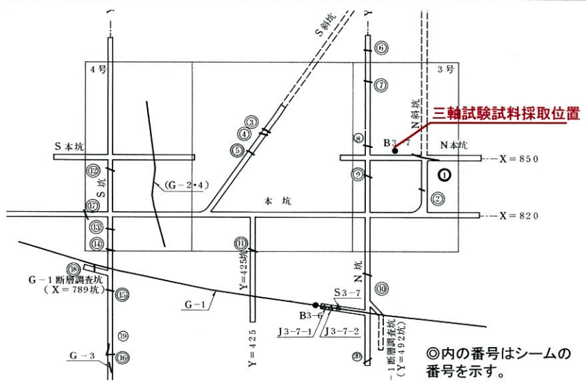
シーム試料採取位置図
