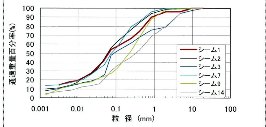
粒径加積曲線
