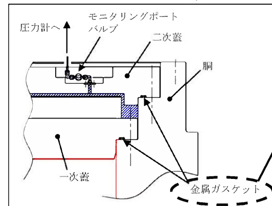
<蓋部詳細図>
