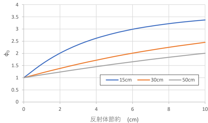
図 C-1 \phi_0 の値 (各炉心長について反射体節約依存性)
